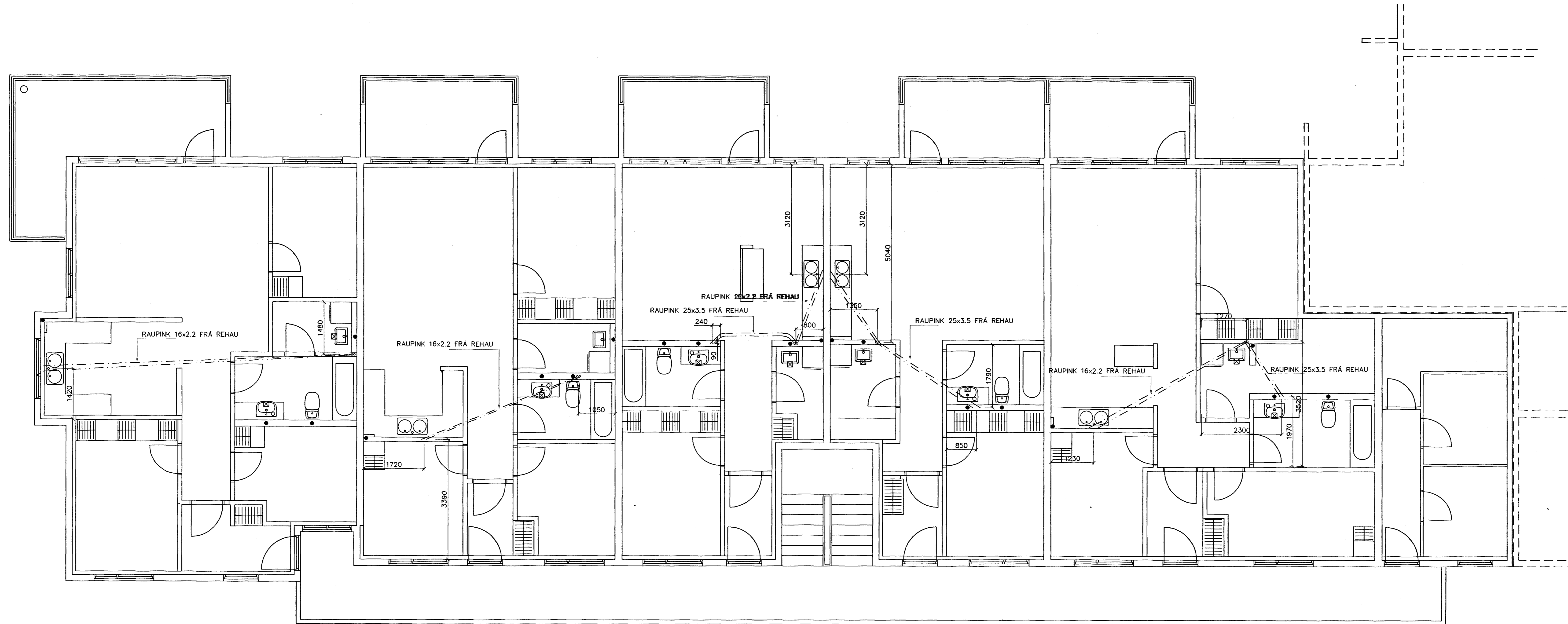
GRUNNMYND 3 HÆÐAR 1:50
