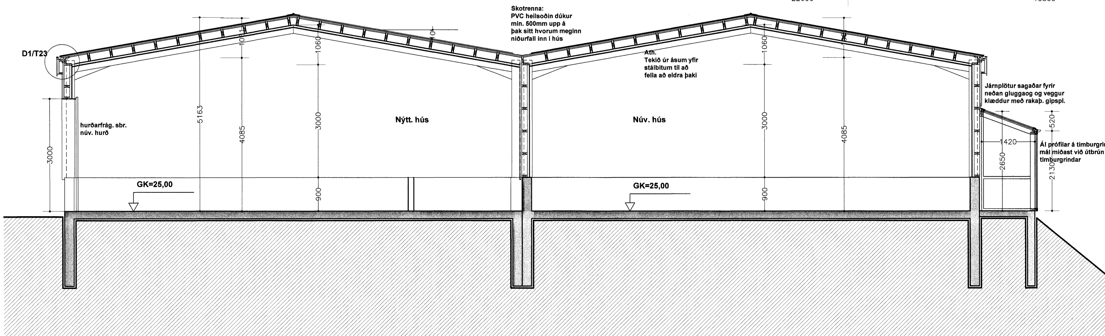
snið B-B
