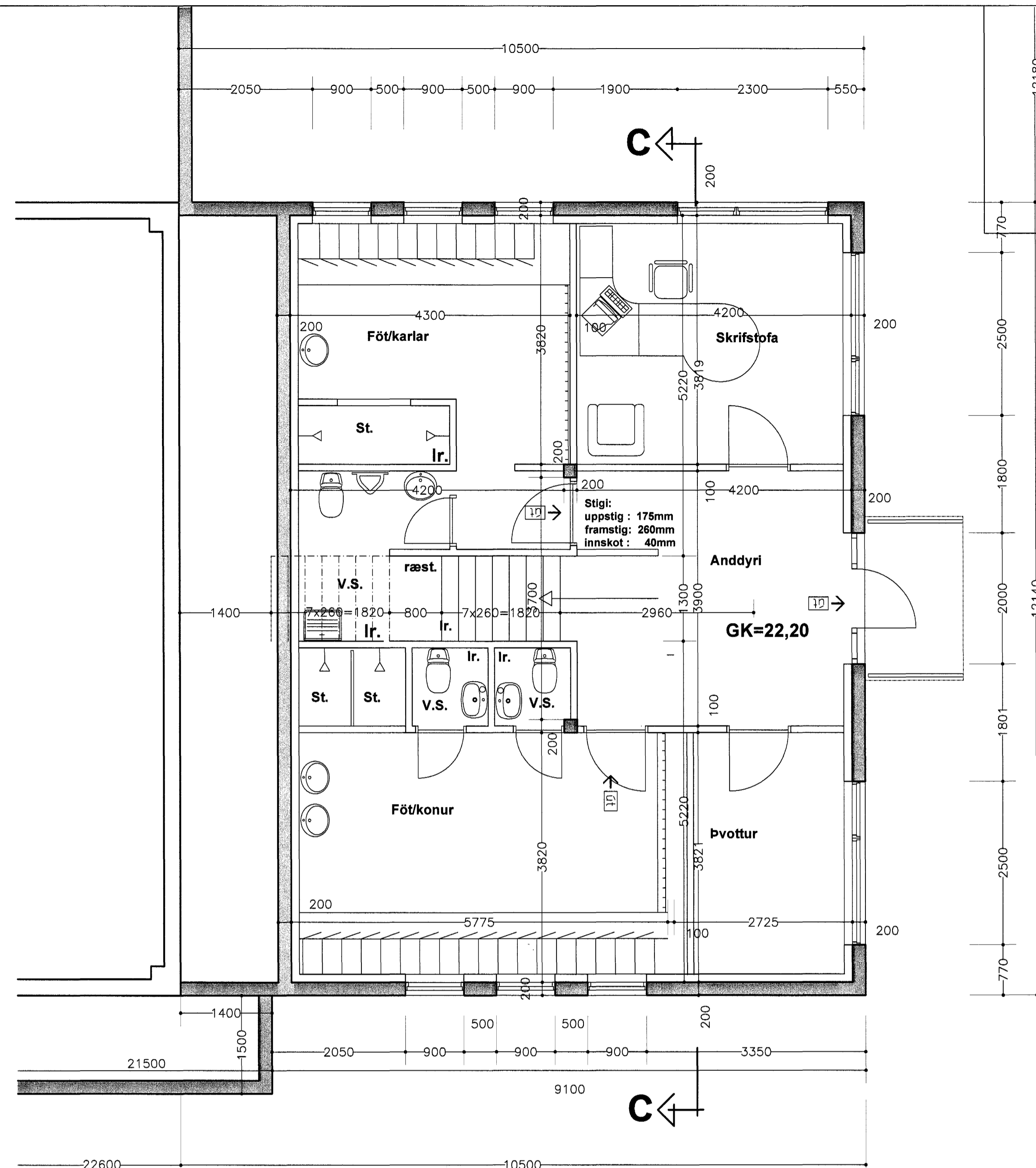
Grunnmynd 1. hæð
