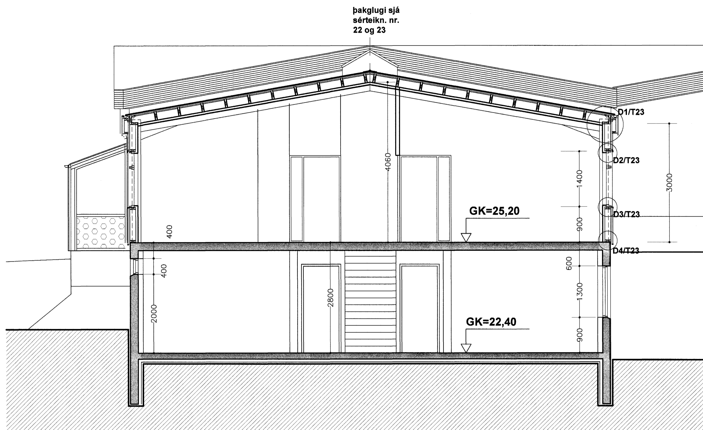
snið C-C
