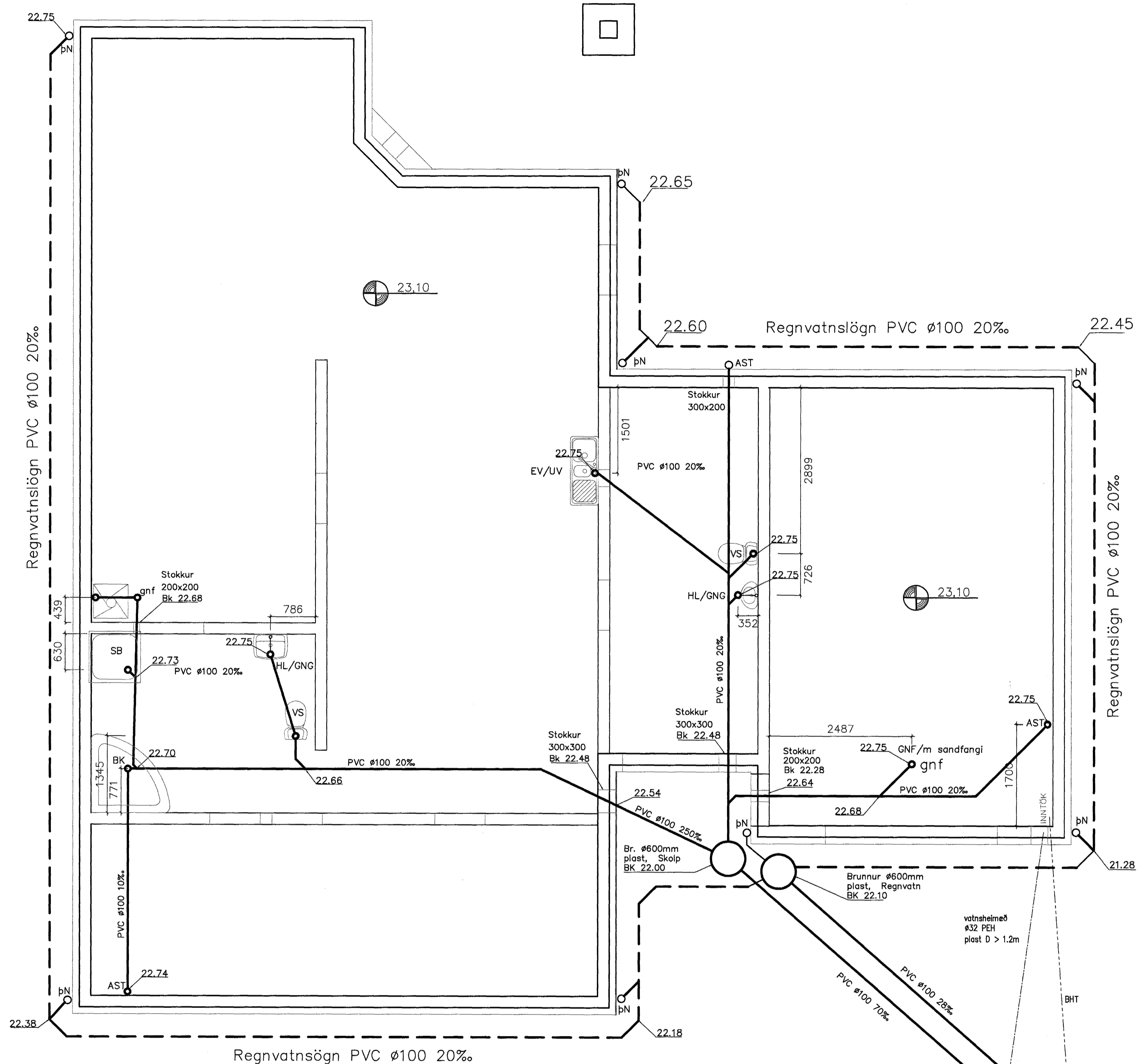
FRÁRENNSLI, GRUNNMYND 1:50
