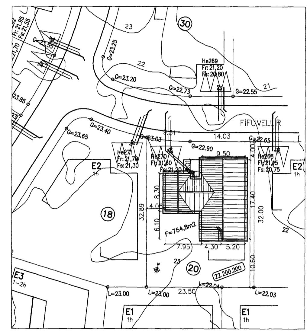
AFSTÖÐUMYND 1:500
