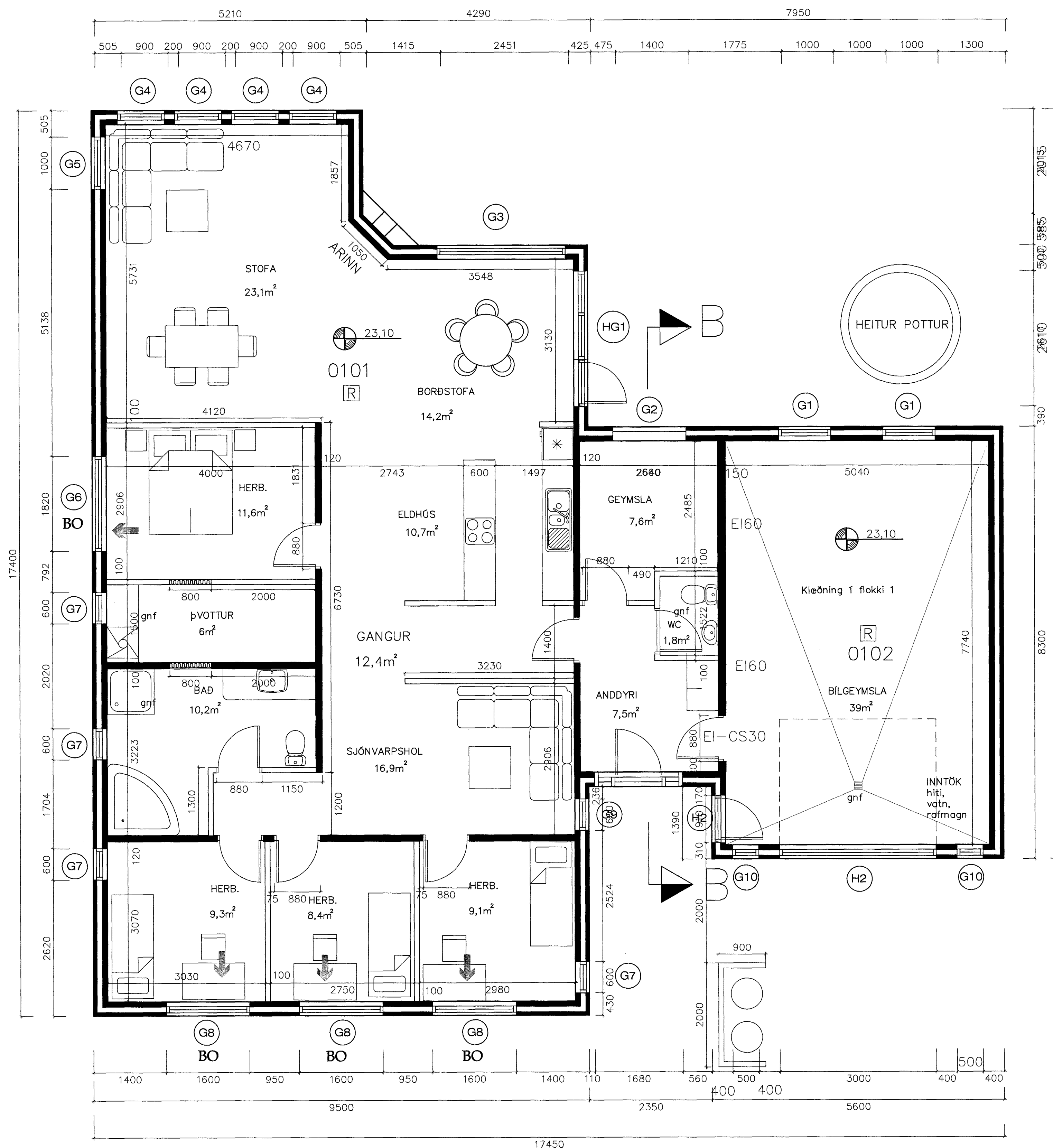
Mkv. 1:50 - GRUNNMYND
