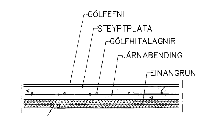
VATNSLAGNIR 20mm FRÁ AquATHERM í DRÁTTARRÖRI
