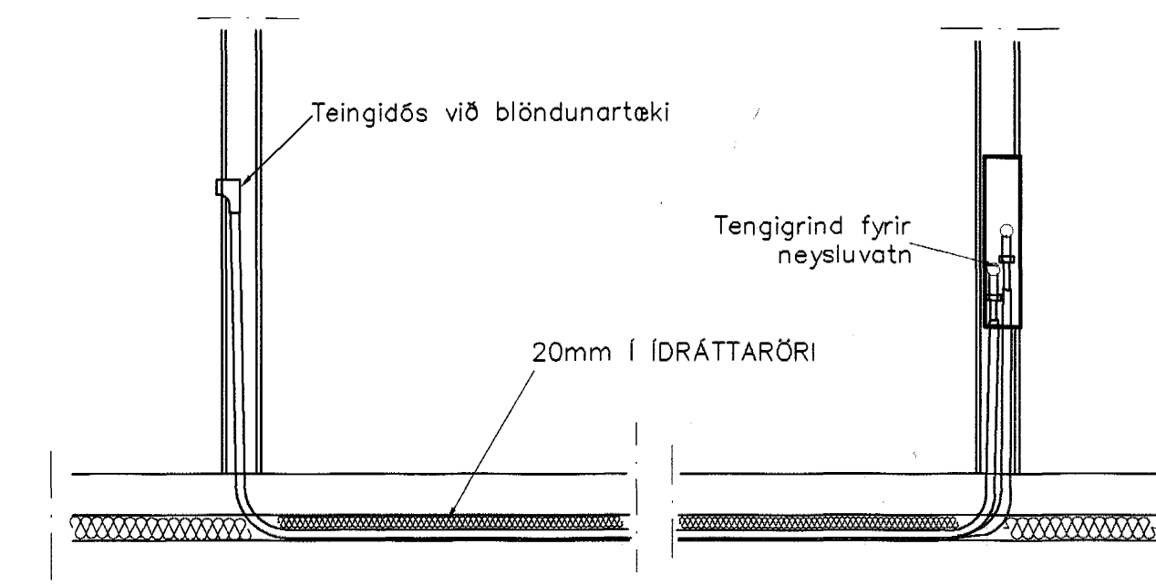
TENING NEYSLUVATNSLAGNA 1:20
