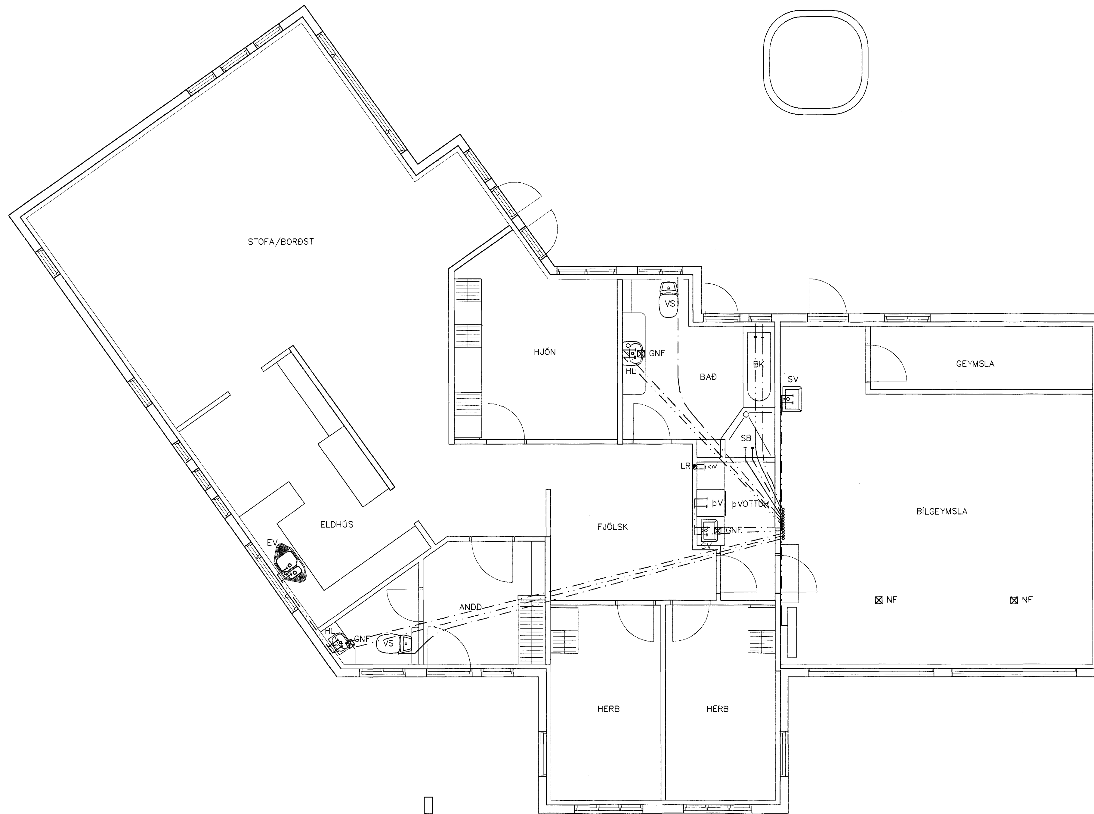
GRUNNMYND 1:50
