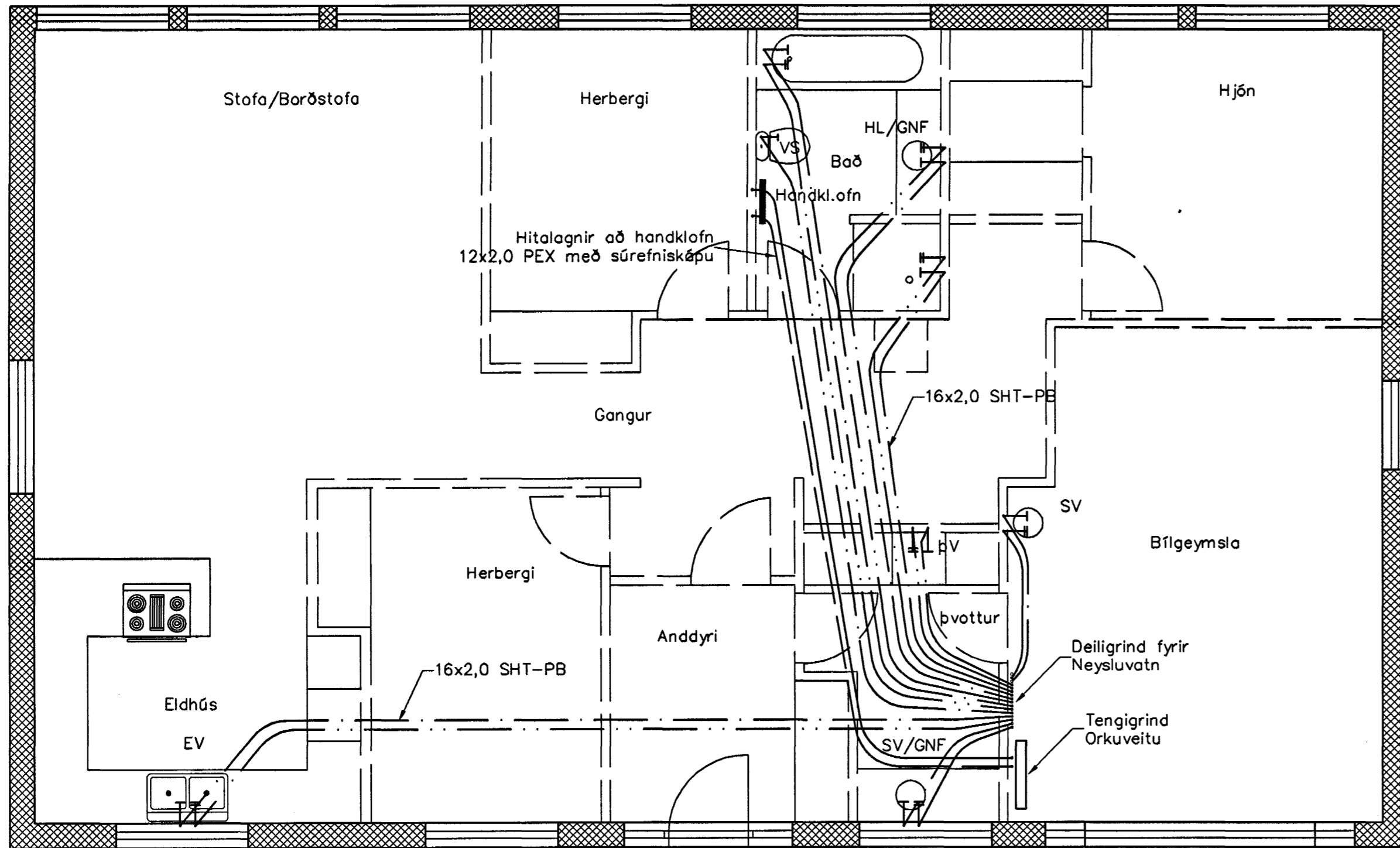
Neysluvatnslagnir, 1:50
