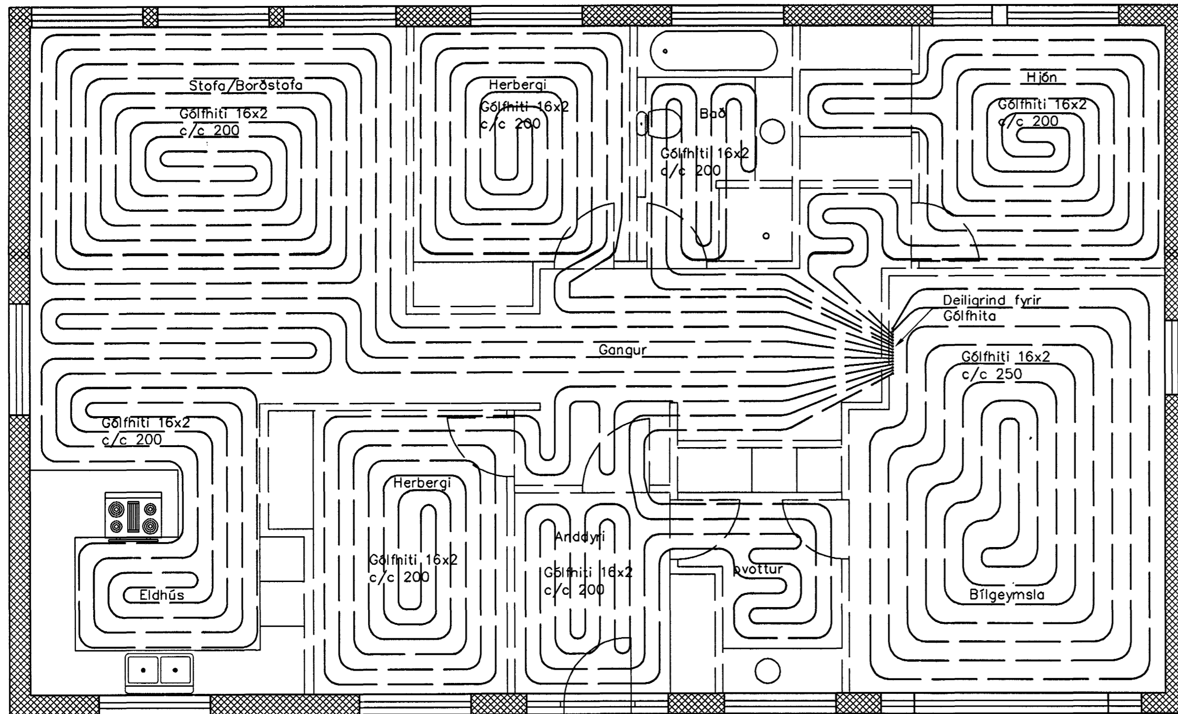
Gólfhitalagnir, 1:50
