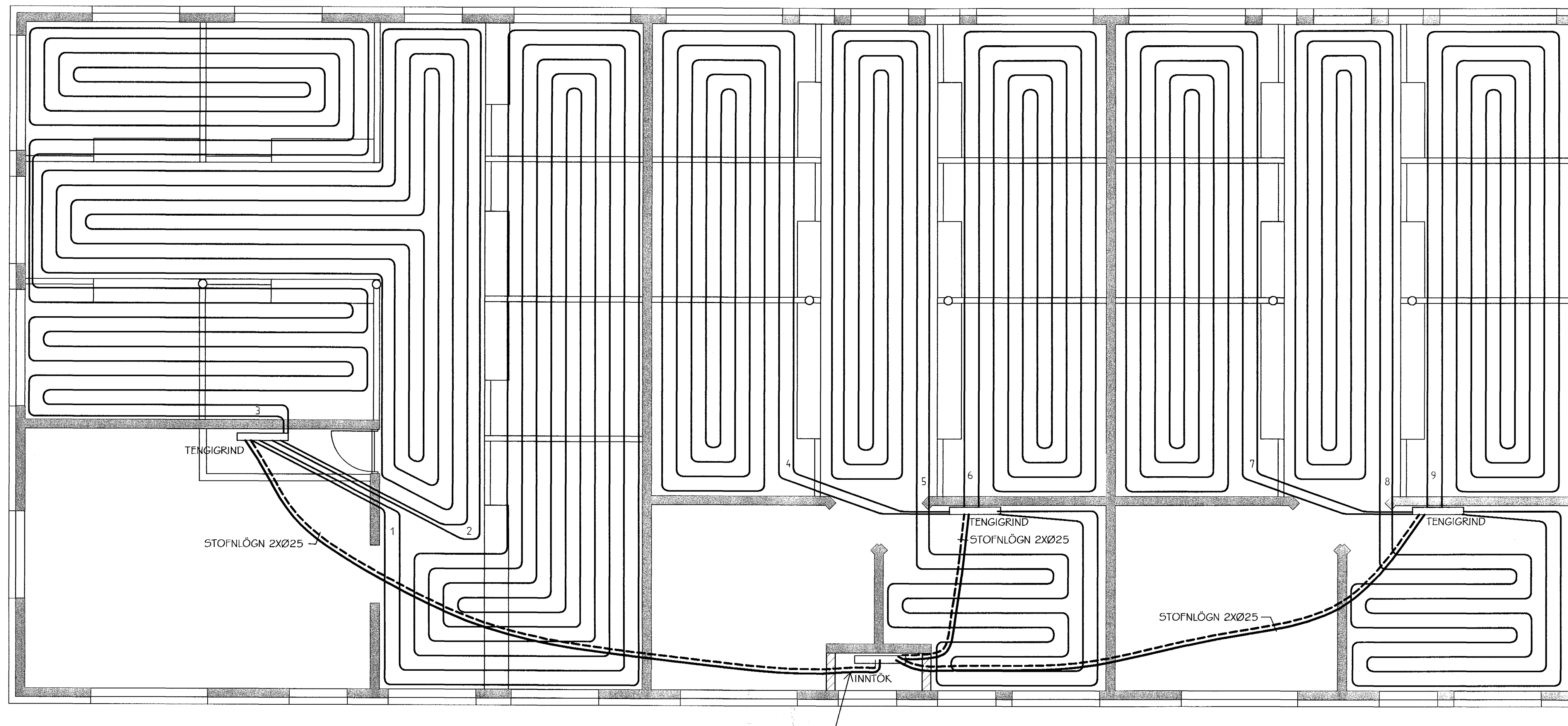
GÓLFHITALAGNIR - GRUNNMYND MKV. 1:50
