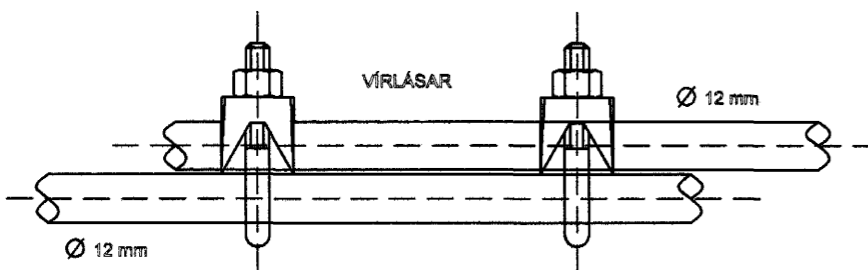
SAMTENGING STEIPUTEINA SETJA SKAL TVO VIRLÁSA Á HVER SAMSEYTI.
