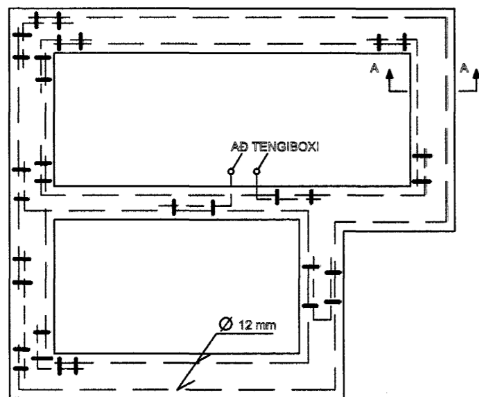
GRUNNMYND SÖKKULVEGGJA
