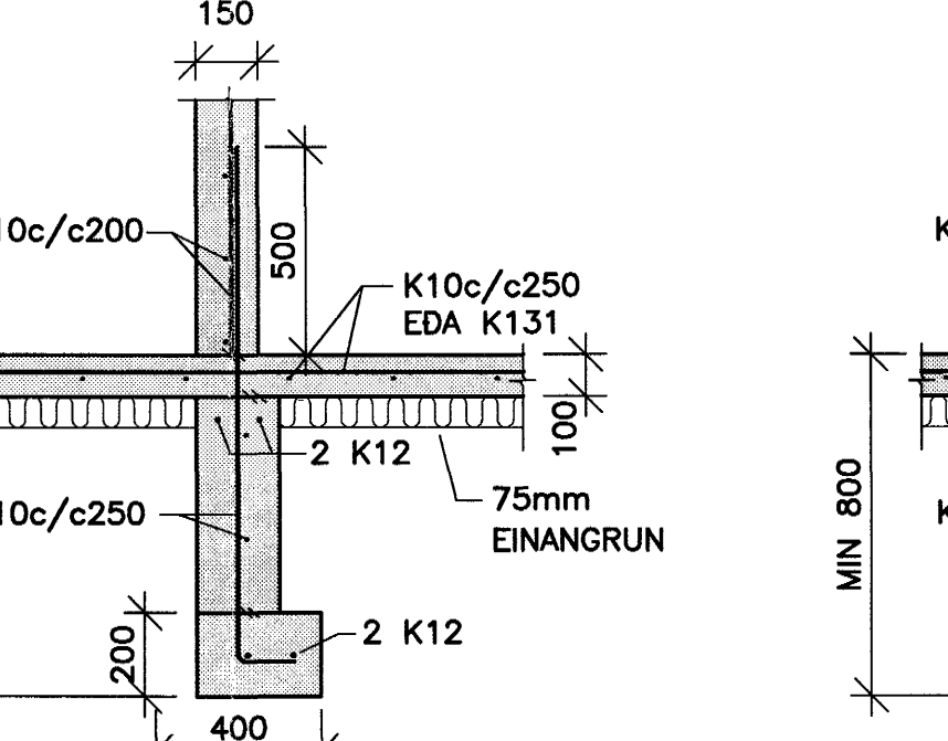
07 SNID 201 1:20
