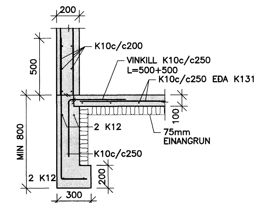
02 SNID 201 1:20
