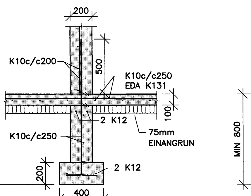
06 SNID 201 1:20
