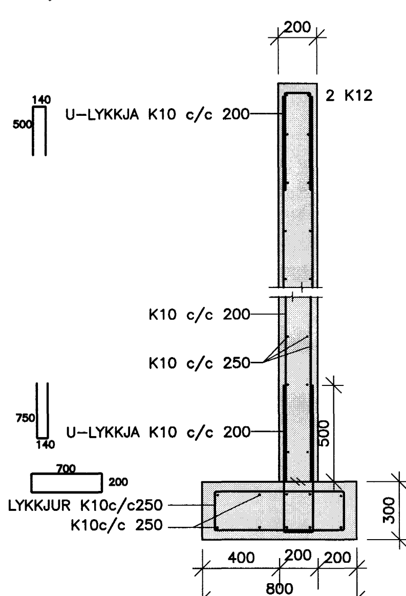
12 SNID 201 1:20
