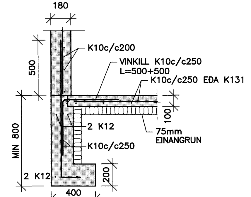
04 SNID 201 1:20
