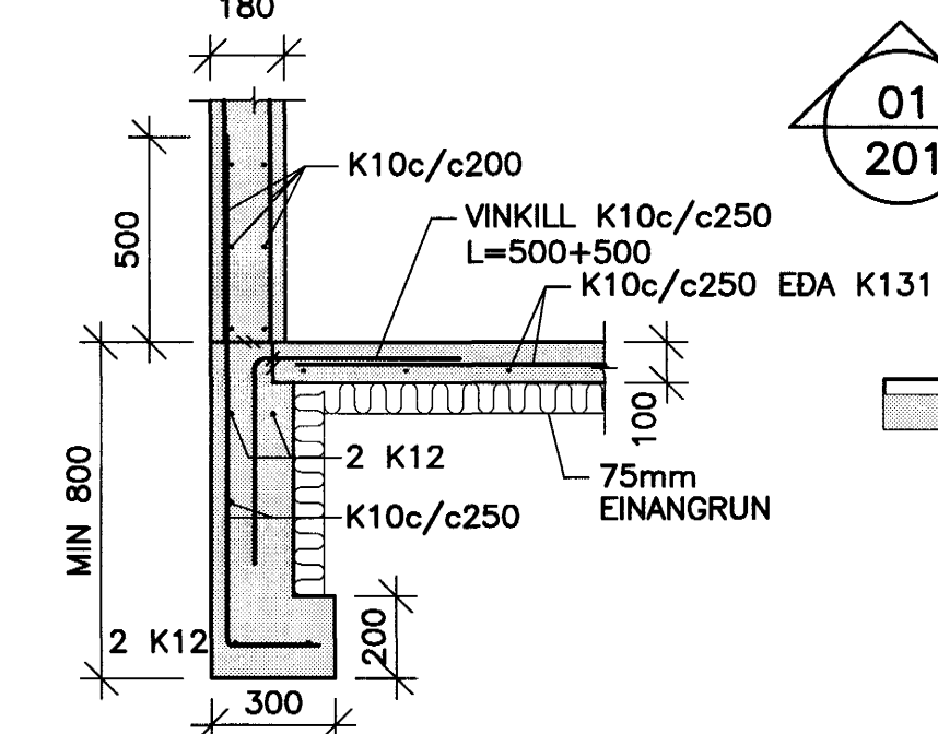
03 SNID 201 1:20
