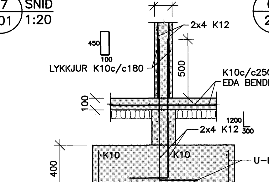
13 SNID 201 1:20
