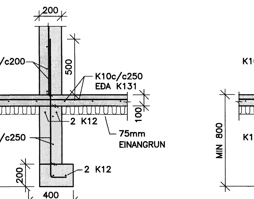
08 SNID 201 1:20
