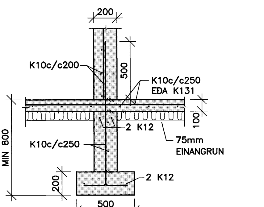
05 SNID 201 1:20
