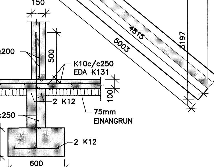
09 SNID 201 1:20
