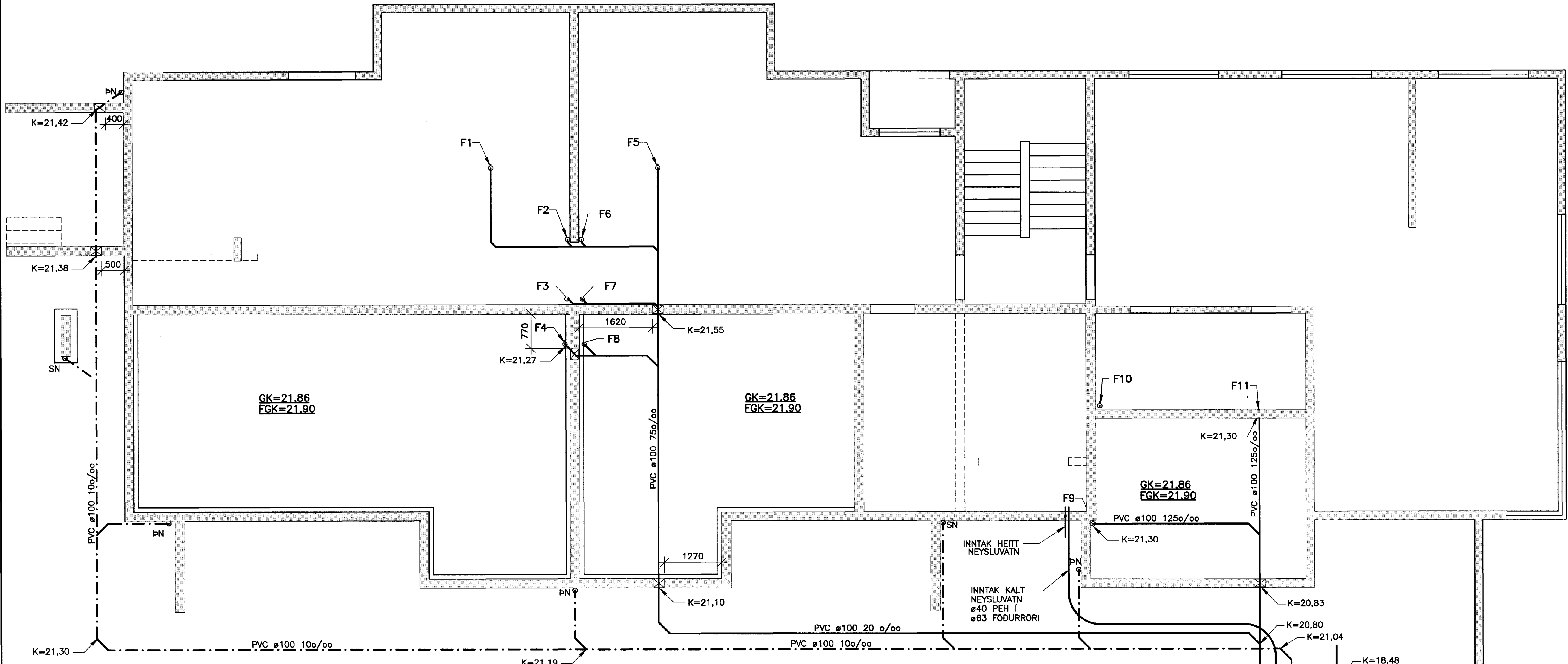
GRUNNLAGNIR GRUNNMYND. 1:50
