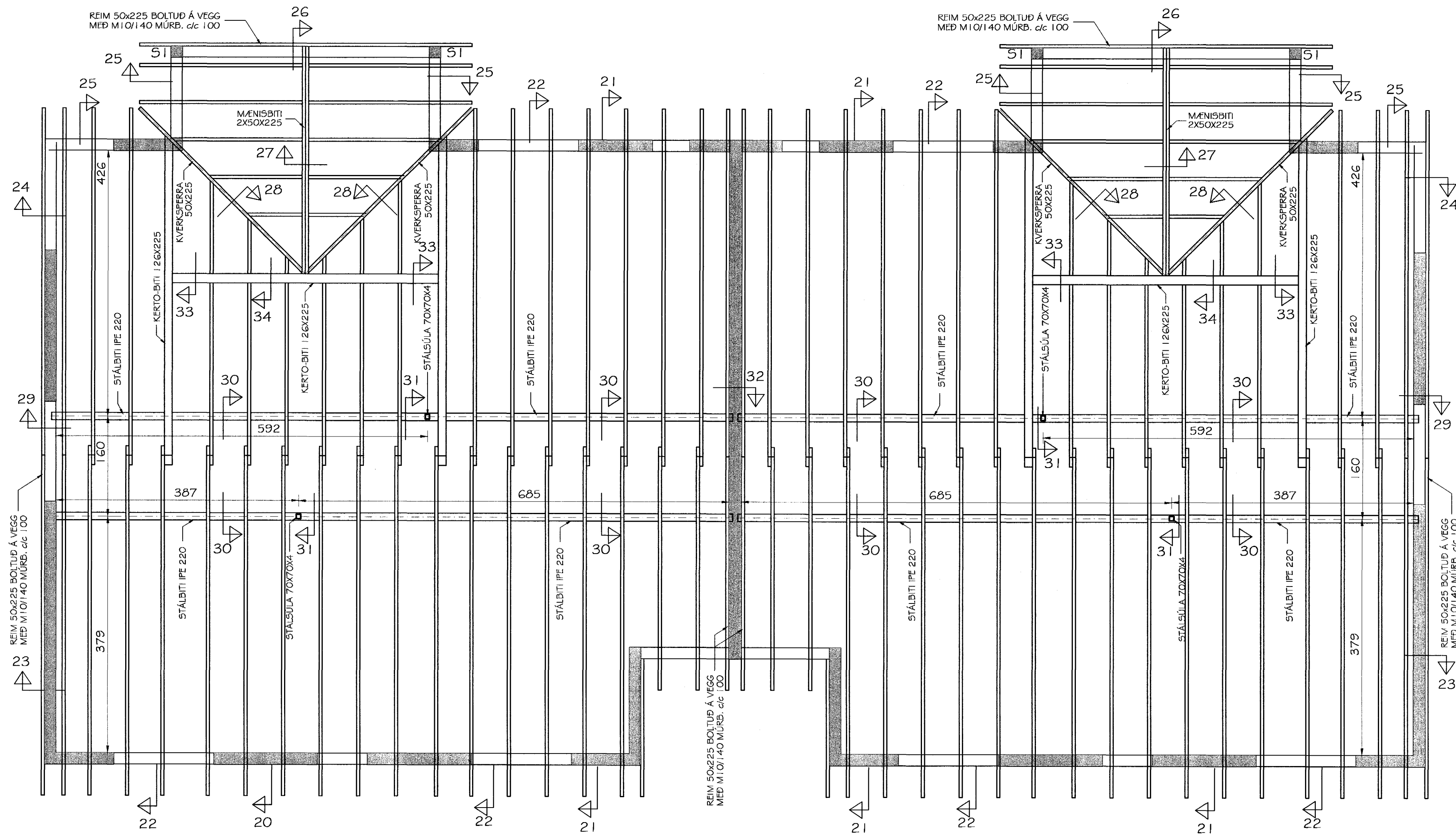
GRUNNMYND ÞAKVIÐA MKV. 1:50
