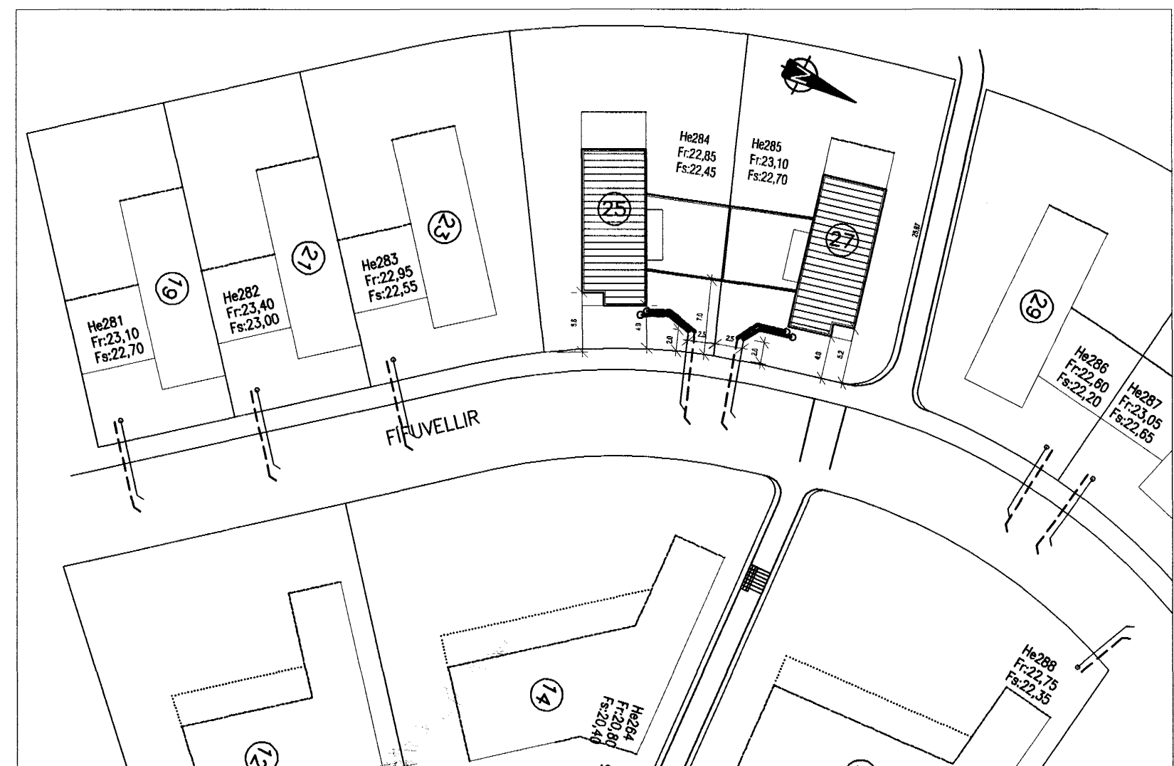
AFSTÖÐUMYND mkv. 1:500
