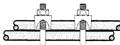
FRÁGANÐUR Á SAMTENGINGUM STEYPUTEINA FYRIR SÖKKULJARSKAUT
