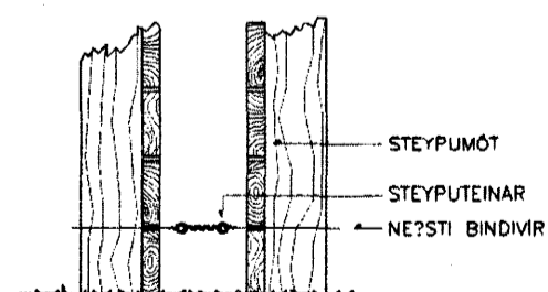
FRÁGANÐUR Á SAMTENGINGUM STEYPUTEINA FYRIR SÖKKULJARSKAUT
