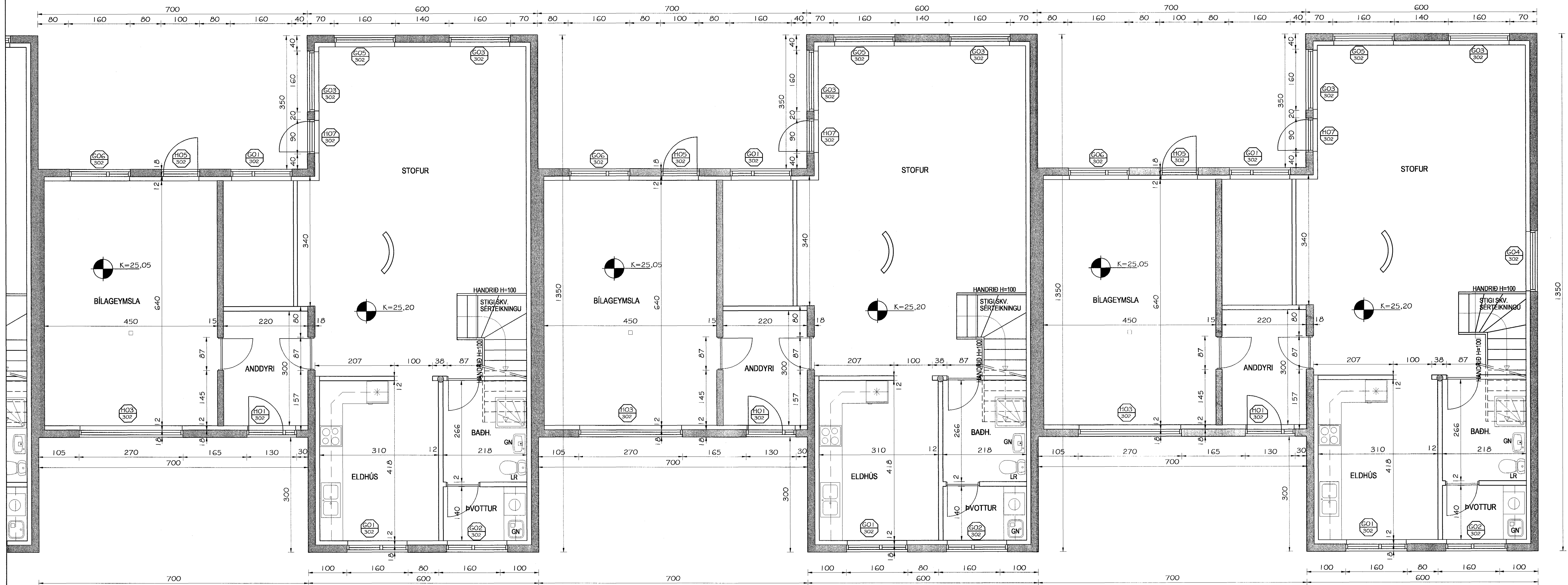
FÍFUVELLIR 19 GRUNNMYND EFRI HÆÐAR MKV. 1:50
