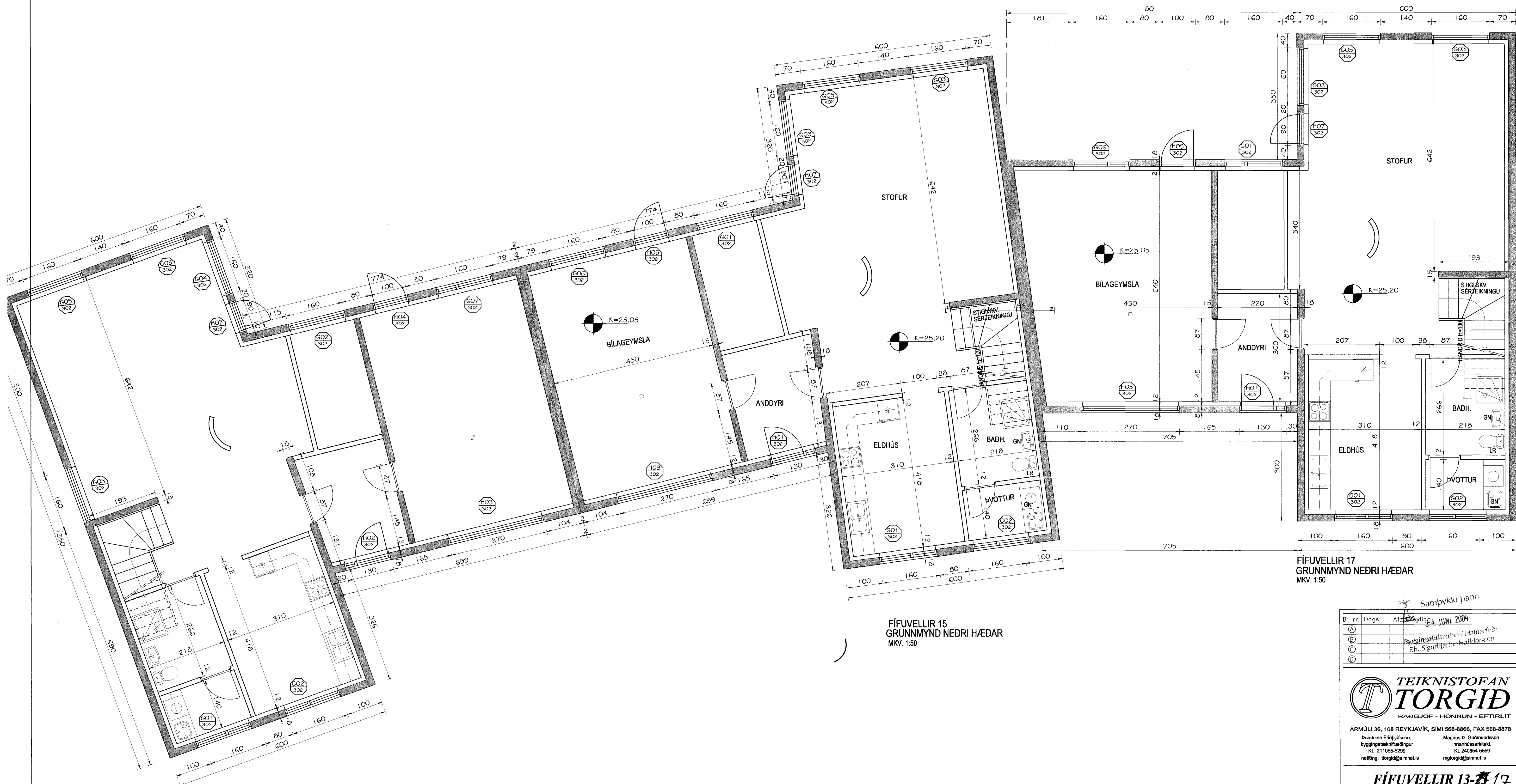
FÍFUVELLIR 13 GRUNNMYND NEDRI HÆÐR MKV. 1:50
