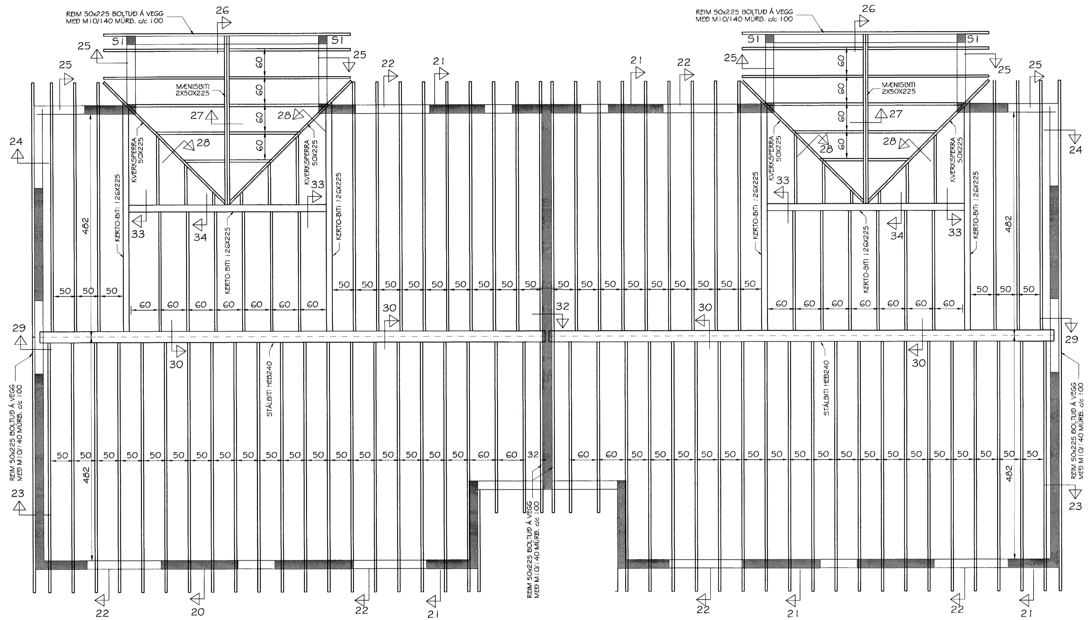
GRUNNMYND PAKVIÐA MKV. 1:50
