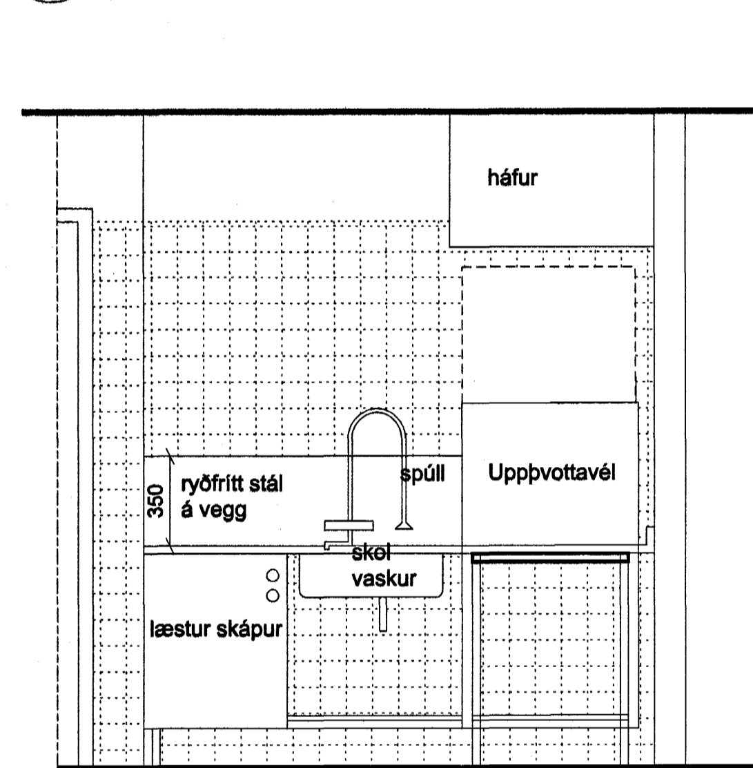
5 70-01 SNEIÐING 1:20
