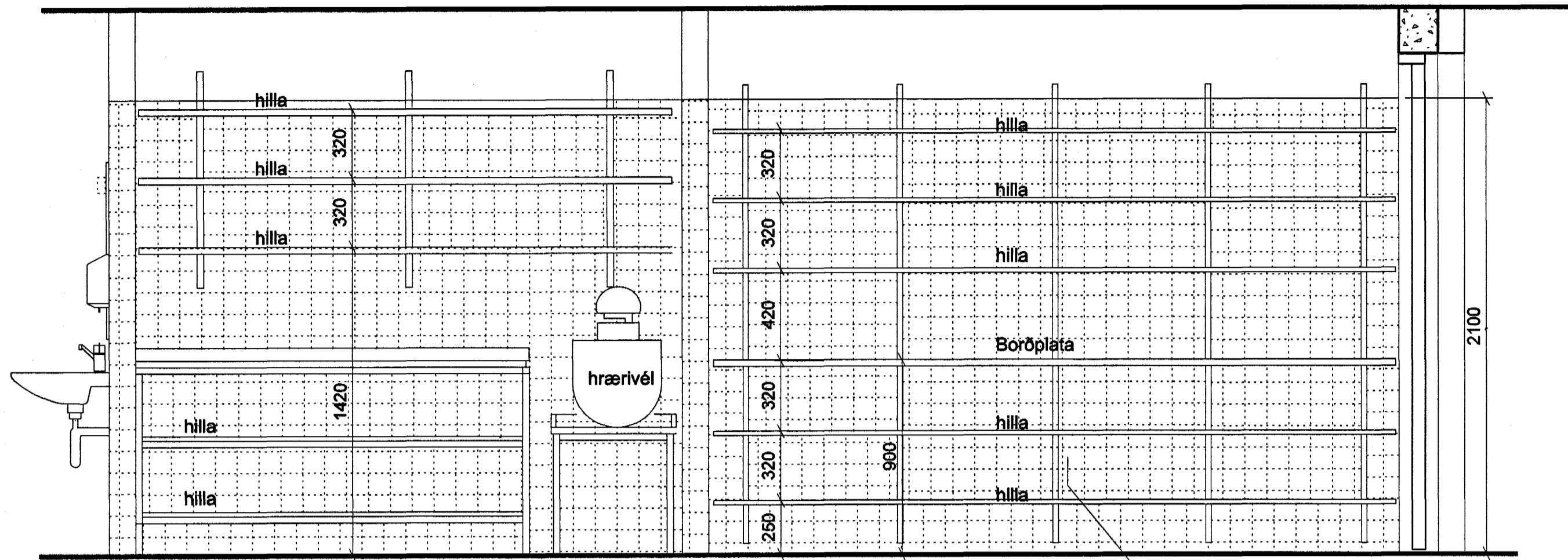
1 70-01 SNEIÐING 1:20
