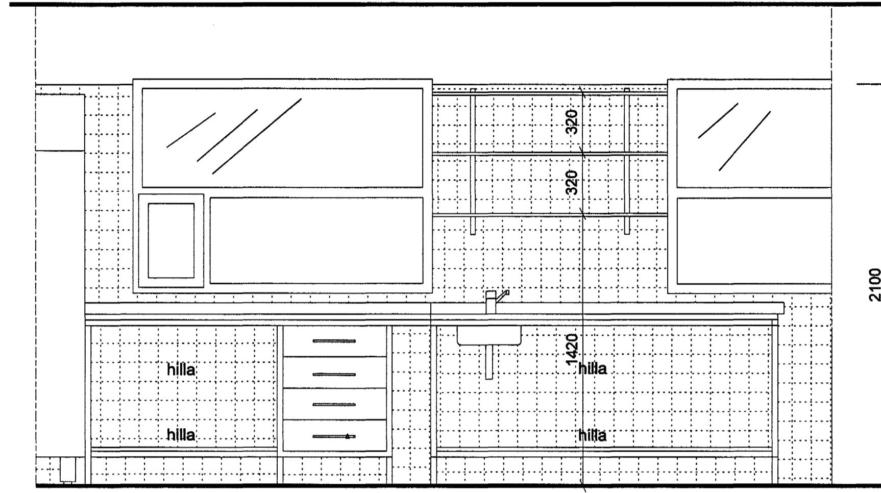
2 70-01 SNEIÐING 1:20
