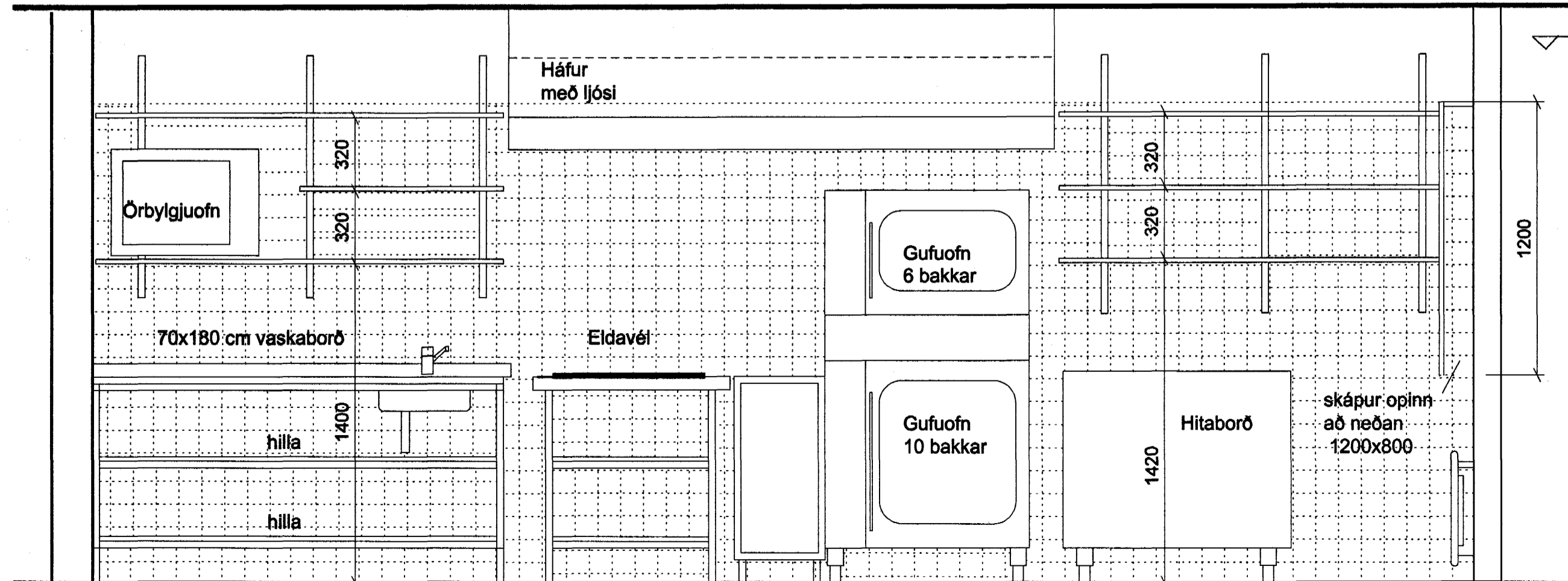
3 70-01 SNEIÐING 1:20
