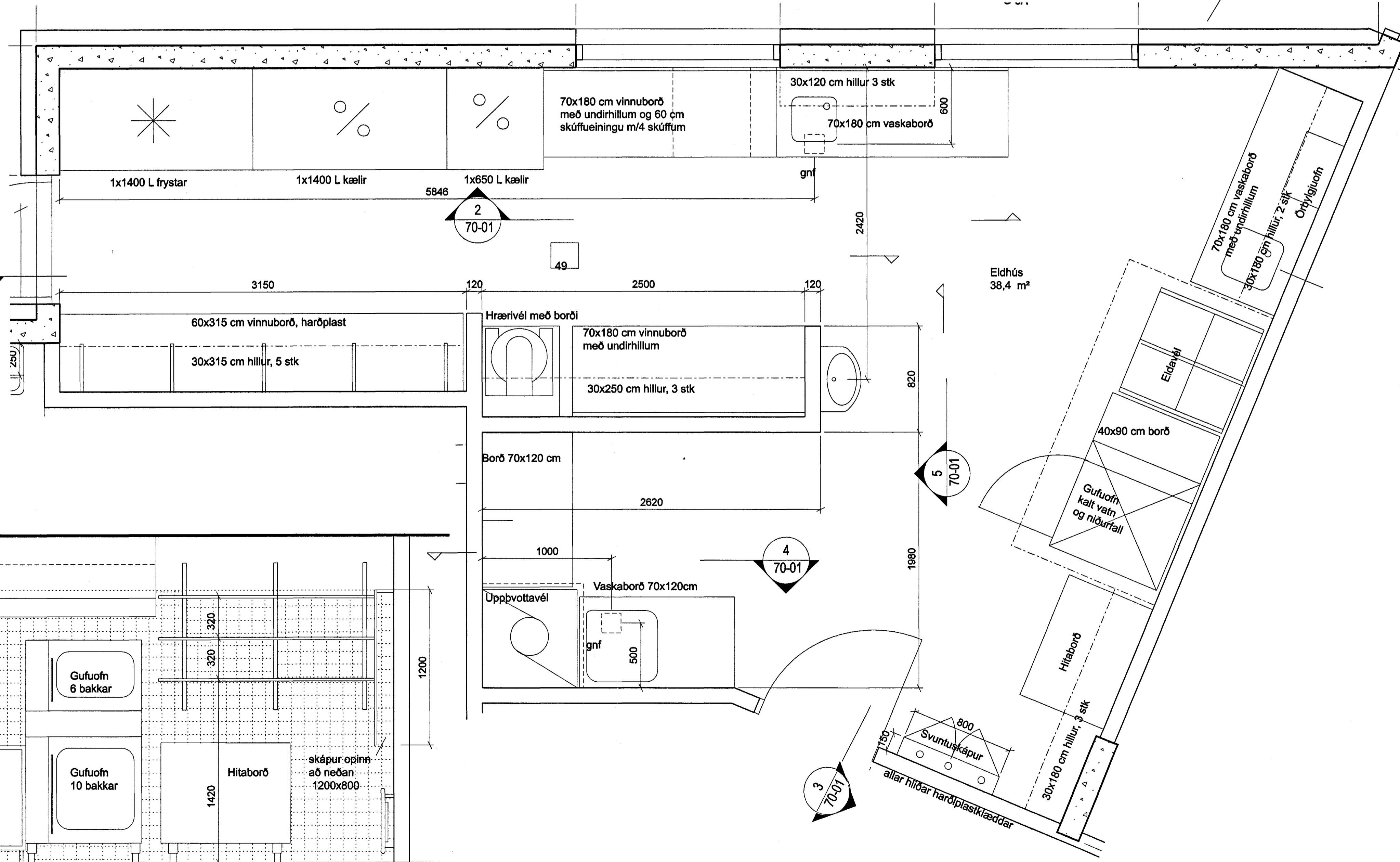
1 70-01 GRUNNMYND 1:20 Eldhús
