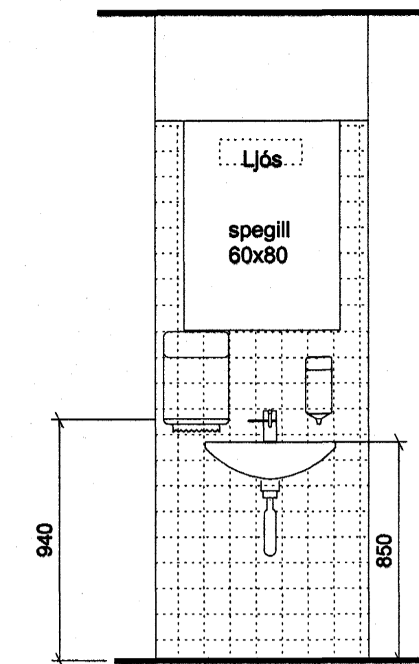
5 70-01 SNEIÐING 1:20
