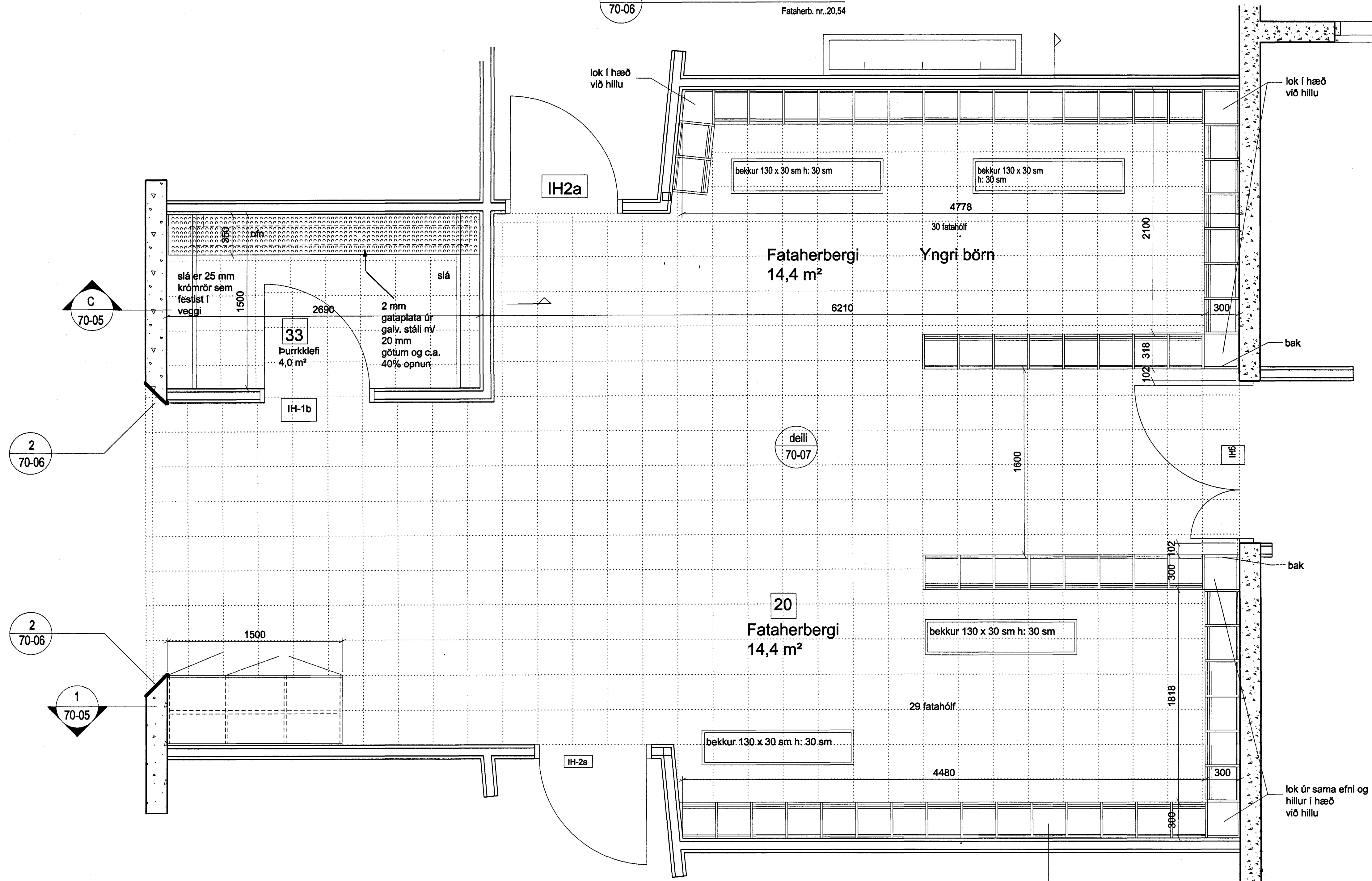
1 20-01 GRUNNMYND 1:20 Fataherb. nr. 20,54
