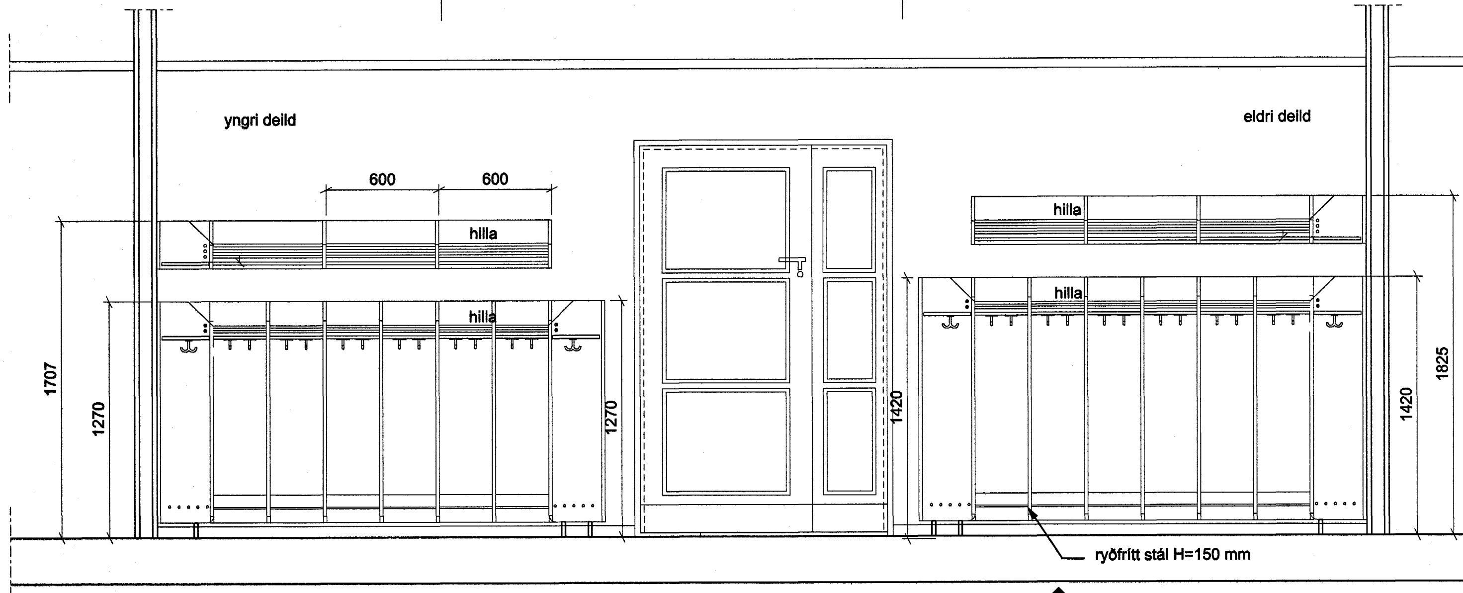
A 70-06 SNEIÐING 1:20 Fataherb. nr. 20,54
