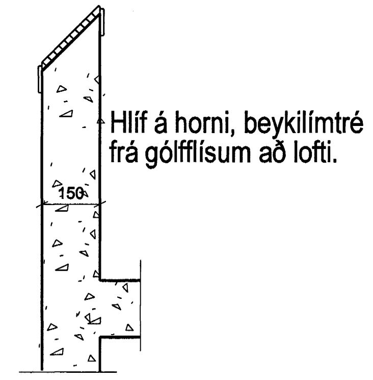
2 70-06 DEILI 1:10 Hlíf á horni á gangi, lárrétt snið
