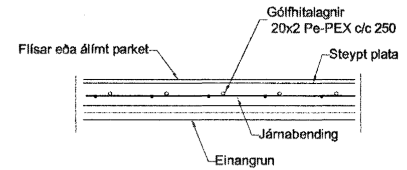
GÓLFHITI SNIÐ, 1:20
