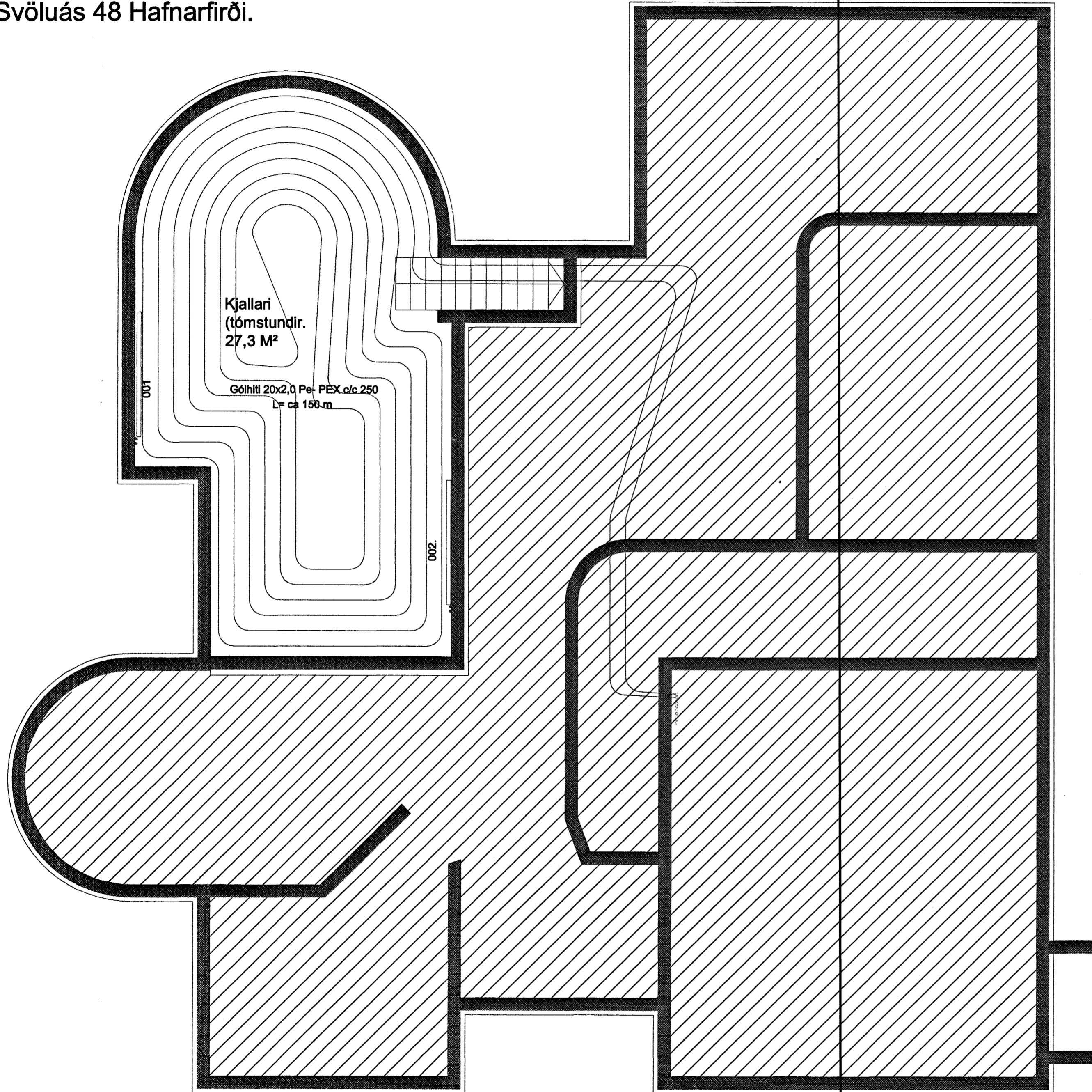
Gólfhiti kjallararými. mkv. 1:50.
