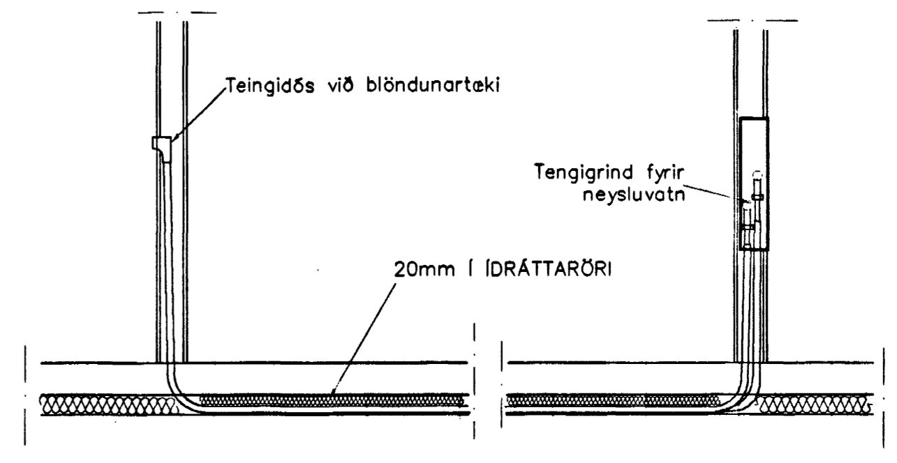
TENGING NEYSLUVATNSLAGNA 1:20
