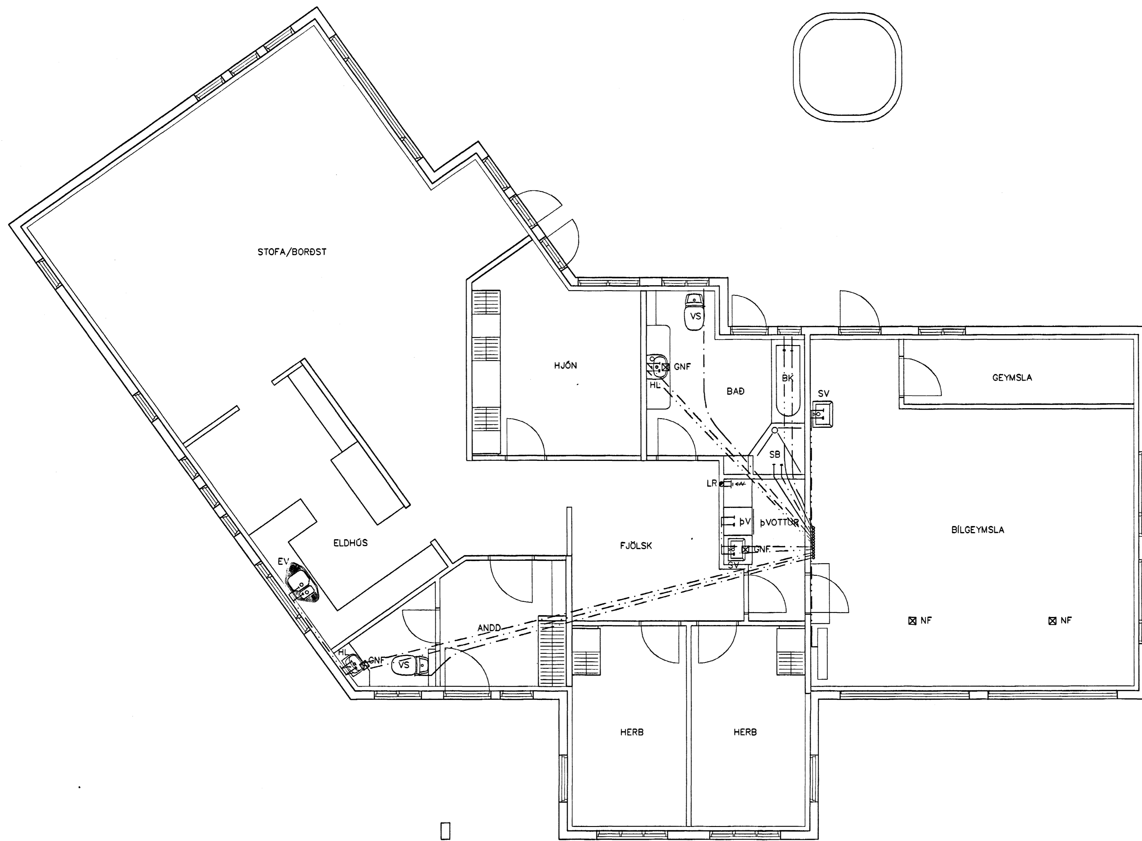
GRUNNMYND 1:50
