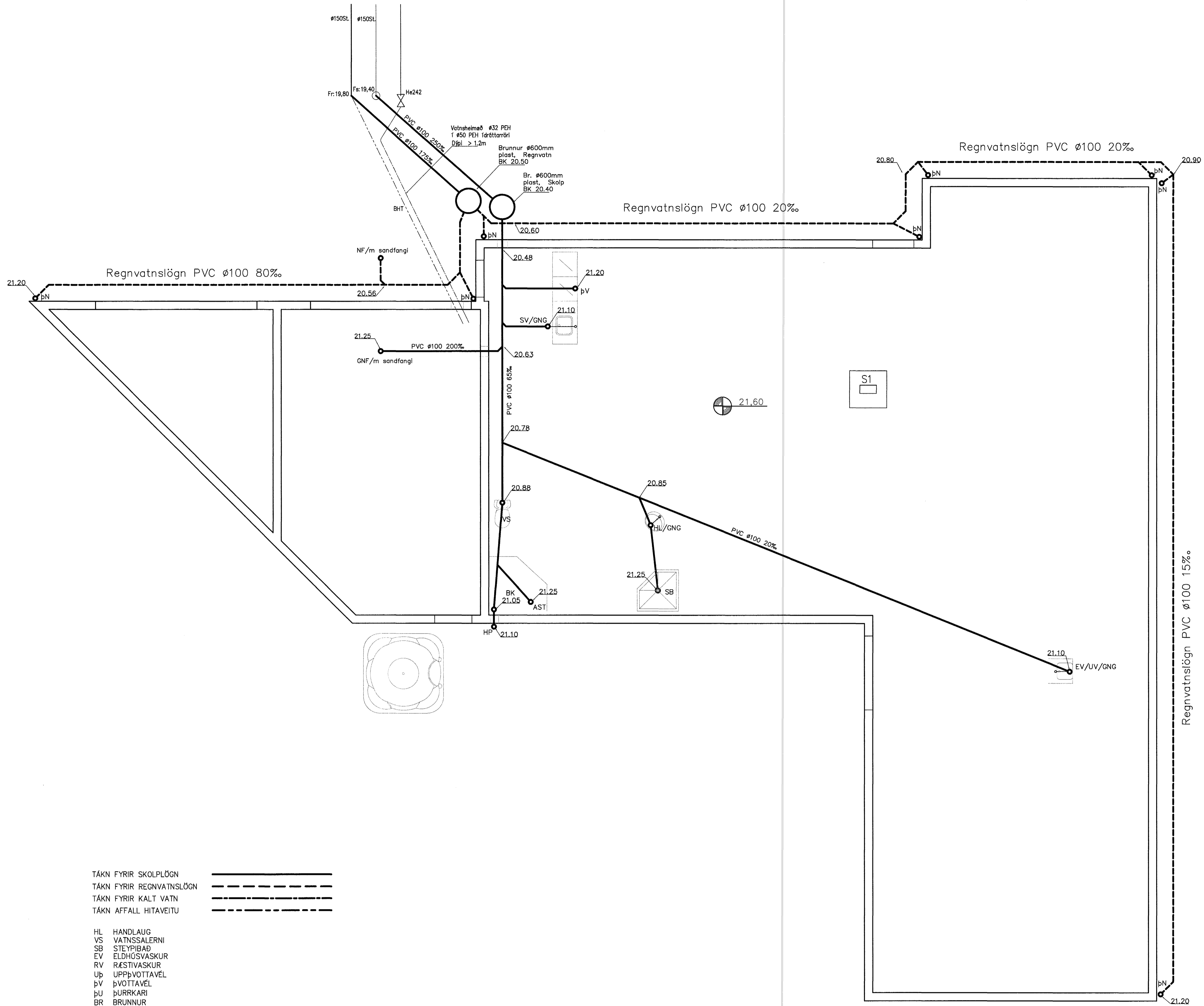
FRÁRENNSLI, GRUNNMYND 1:50
