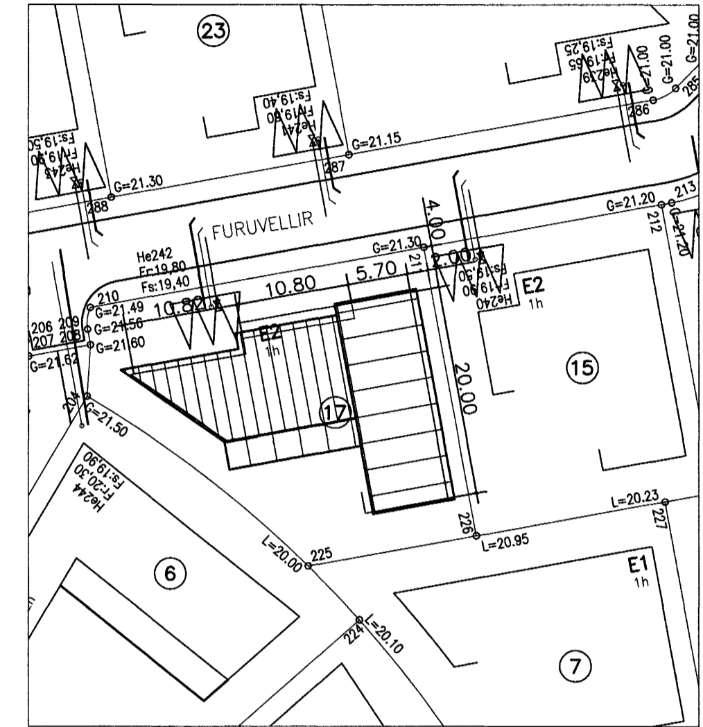
AFSTÖÐUMYND 1:500
