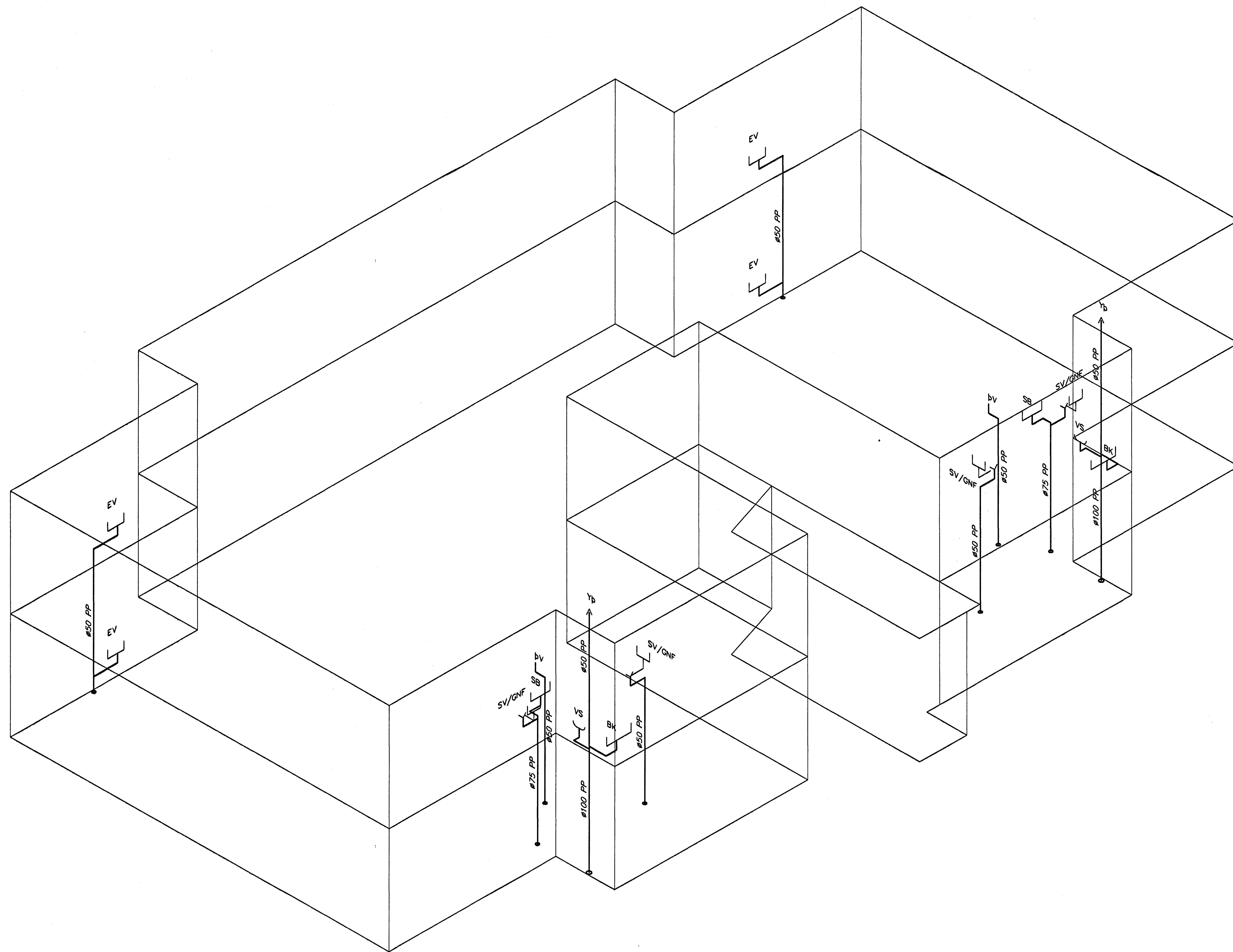
Fráveitulagnir, Rúmmynd, 1:50
