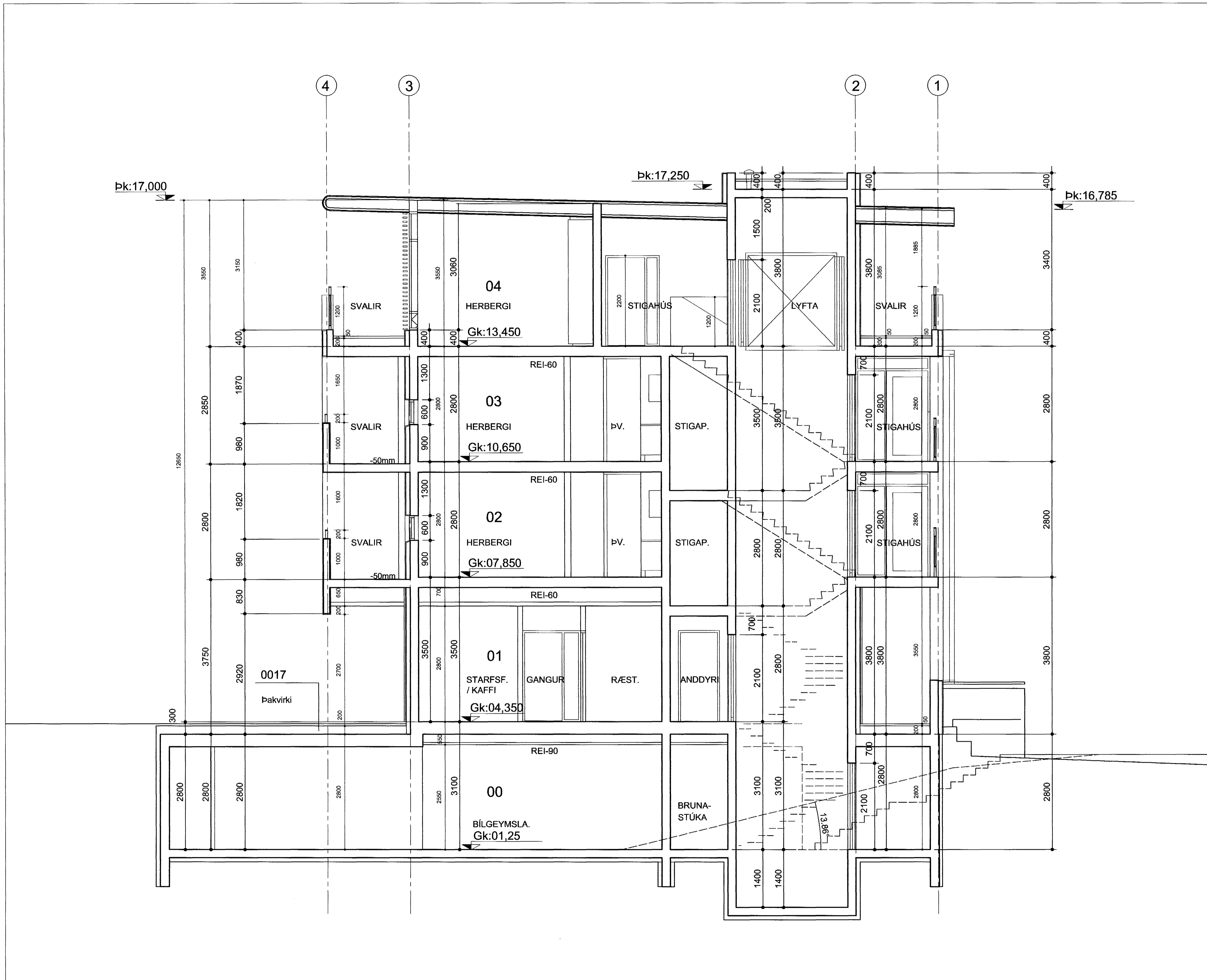
SNEIDING A-A MKV 1:50
