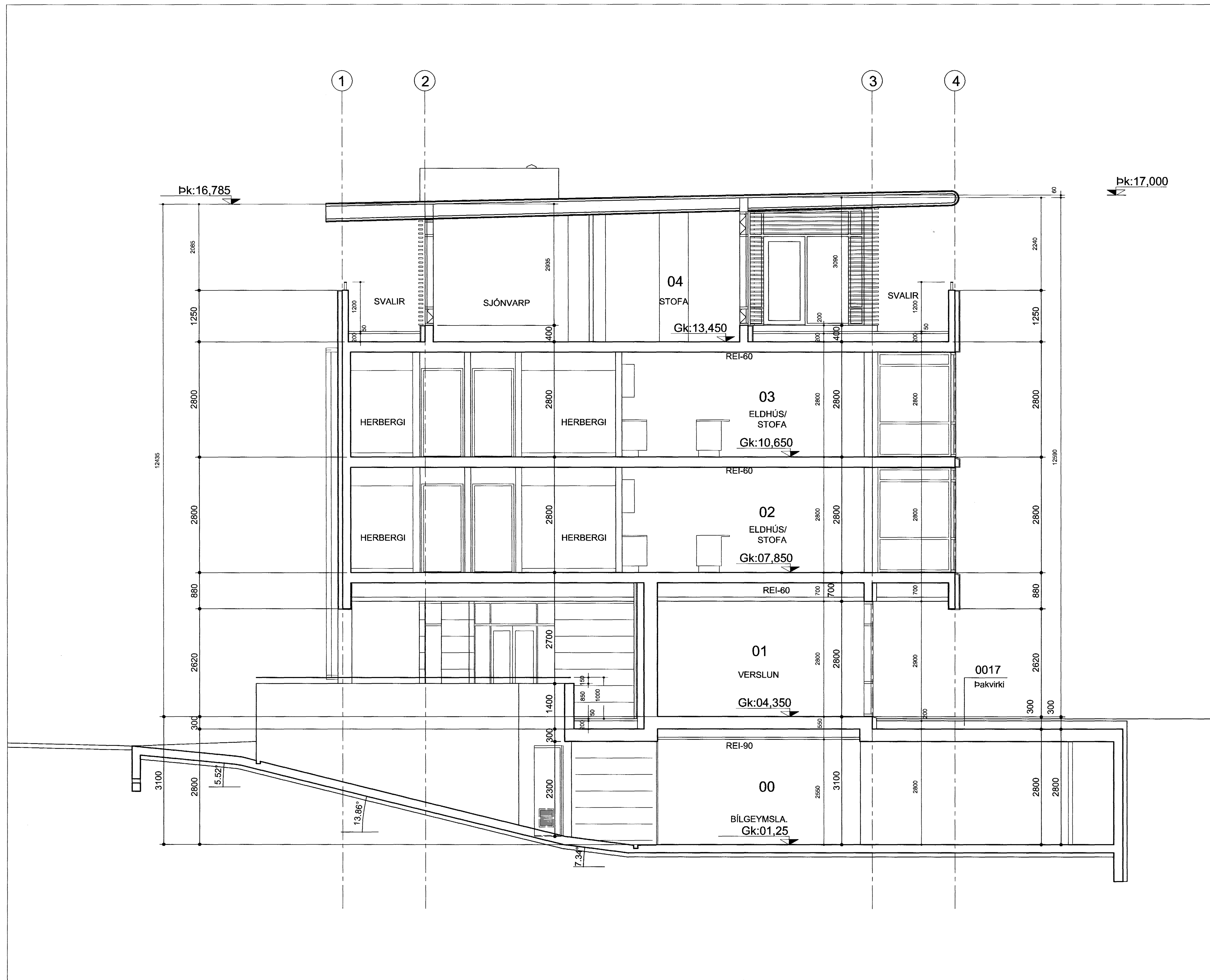
SNEIÐING B-B MKV 1:50
