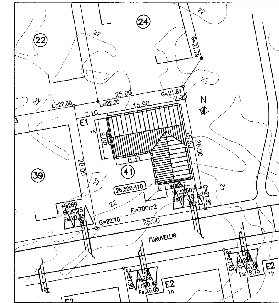
AFSTÖÐUMYND 1:500
