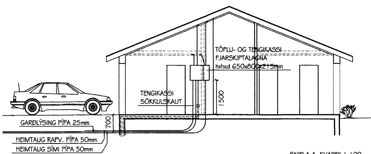
SNID A-A, KVARDI 1:100 Samþykkt þann 05 MAI 2004 Byggingafulltrúinn í Hafnarfirði F.h. Sigurbjartur Halldórsson
