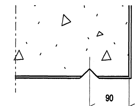
Droprauf 25x25 mm, þríkantlíst í steypu
