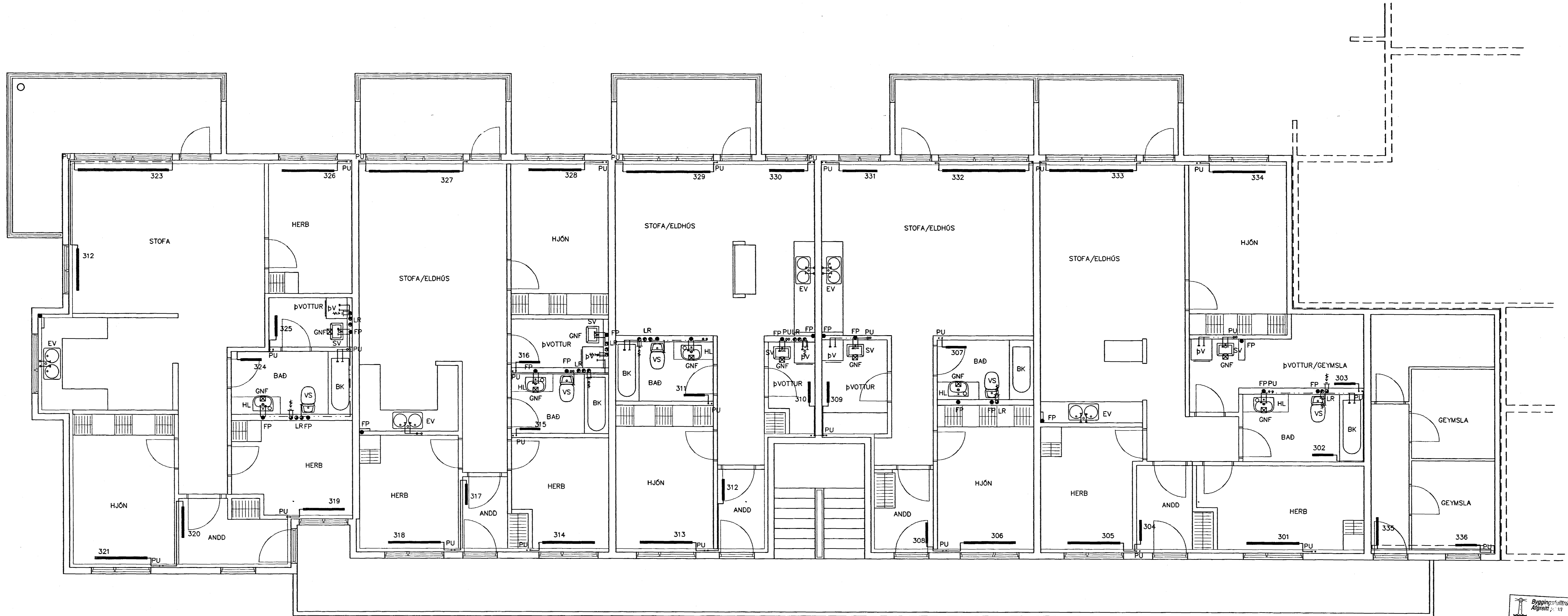
GRUNNMYND 3 HÆÐAR 1:50
