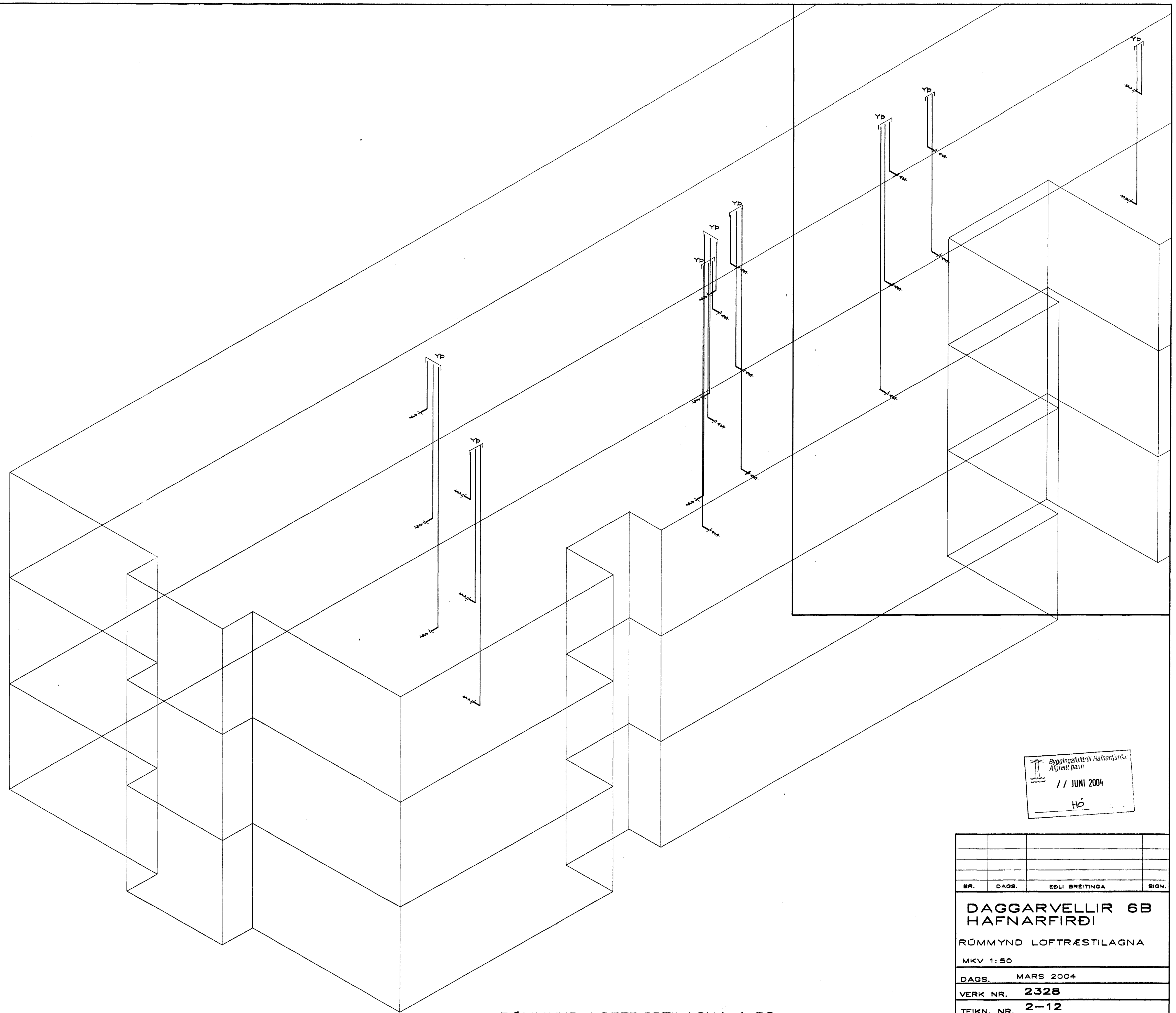
RÚMMYND LOFTRÆSTILAGNA 1:50
