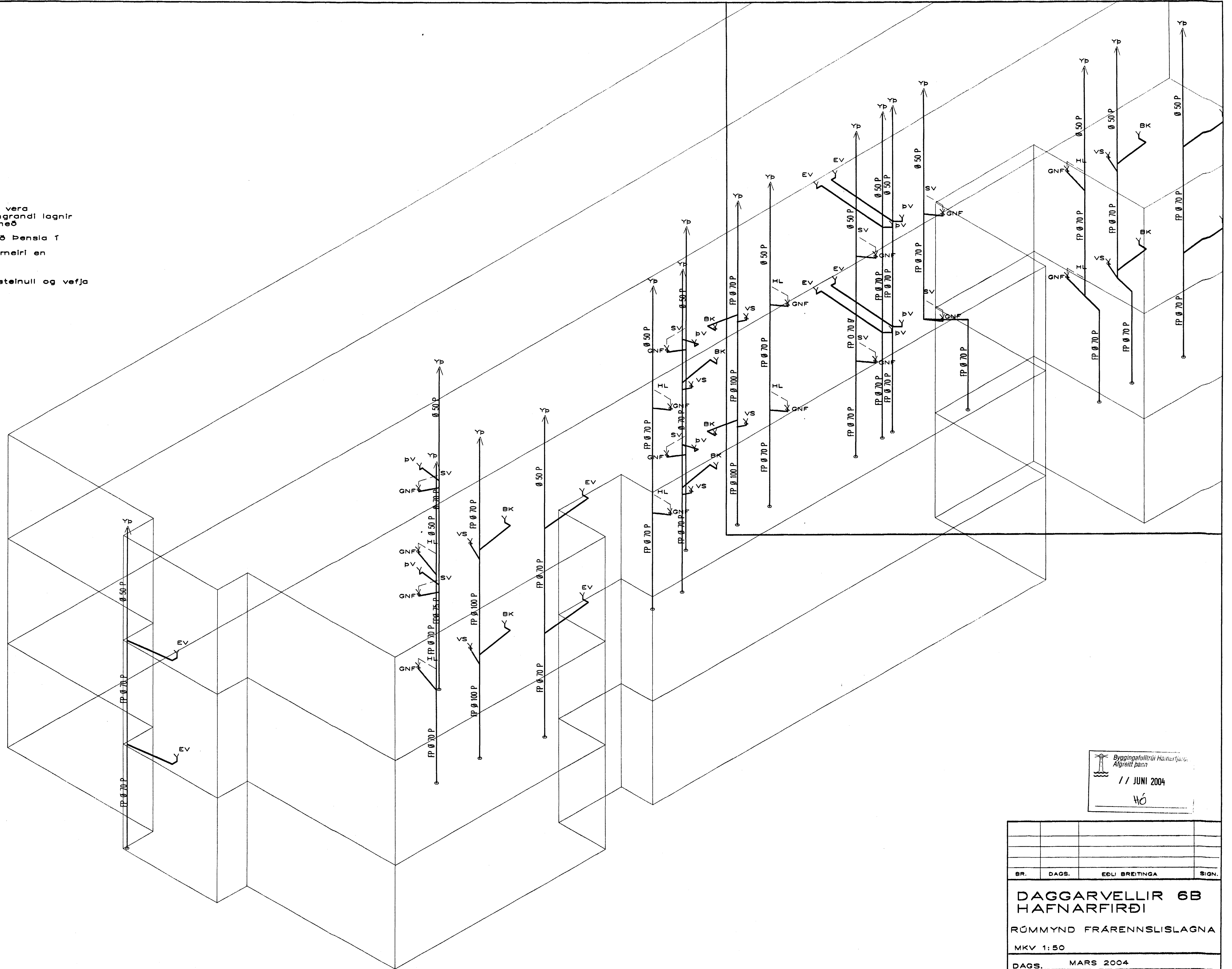
RÚMMYND FRÆRENNSLISLAGNA 1:50
