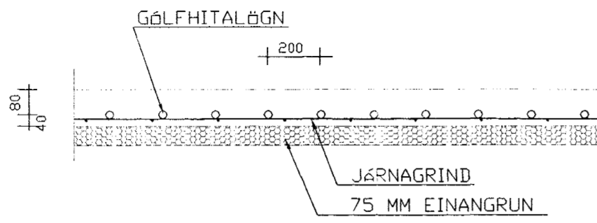
SNID Í GÖLFHITALÖGN 1:20
