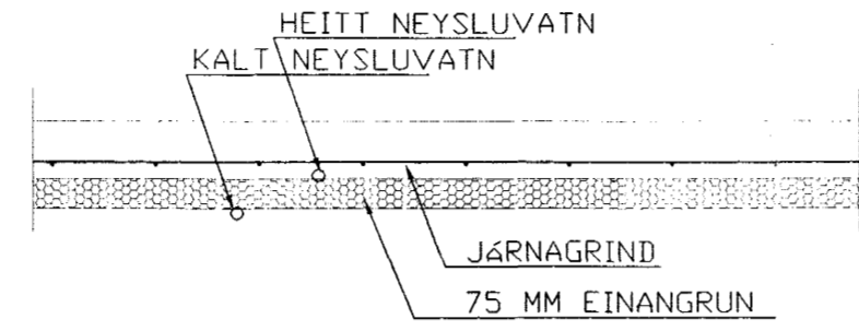
SNID Í NEYSLUVATN, RÖR Í RÖR 1:20
