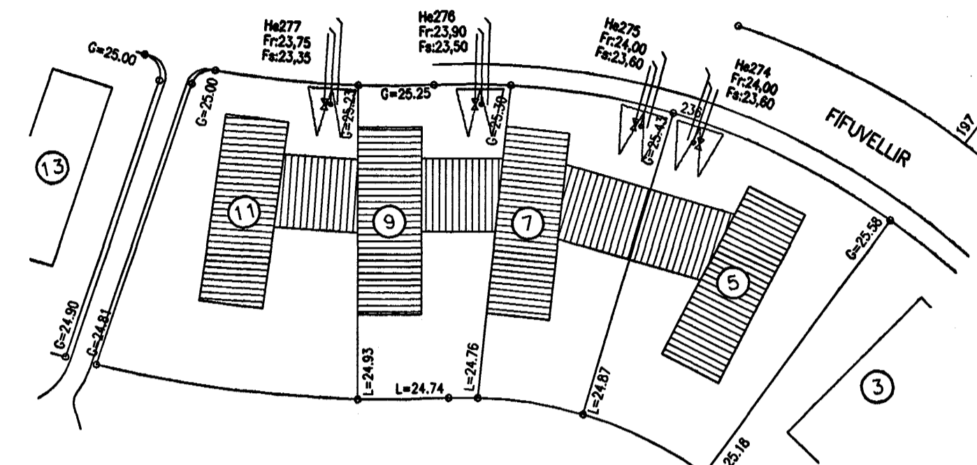
Afstöðumynd, 1:500
