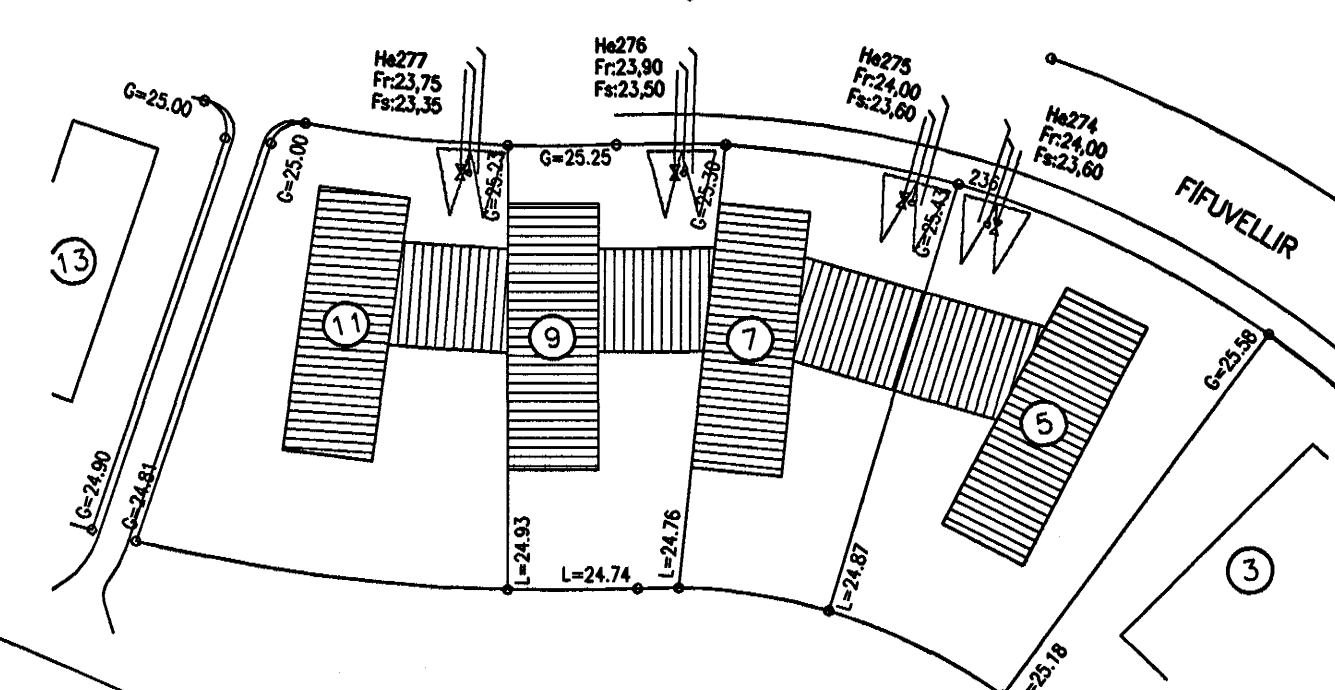
Afstöðumynd, 1:500
