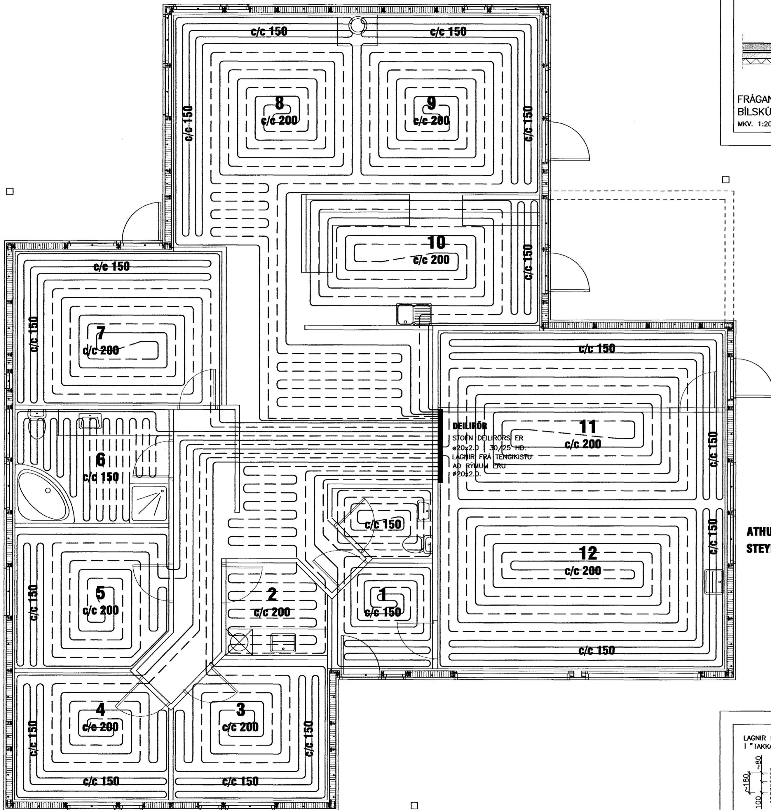
GRUNNMYND HITALAGNA MKV. 1:50
