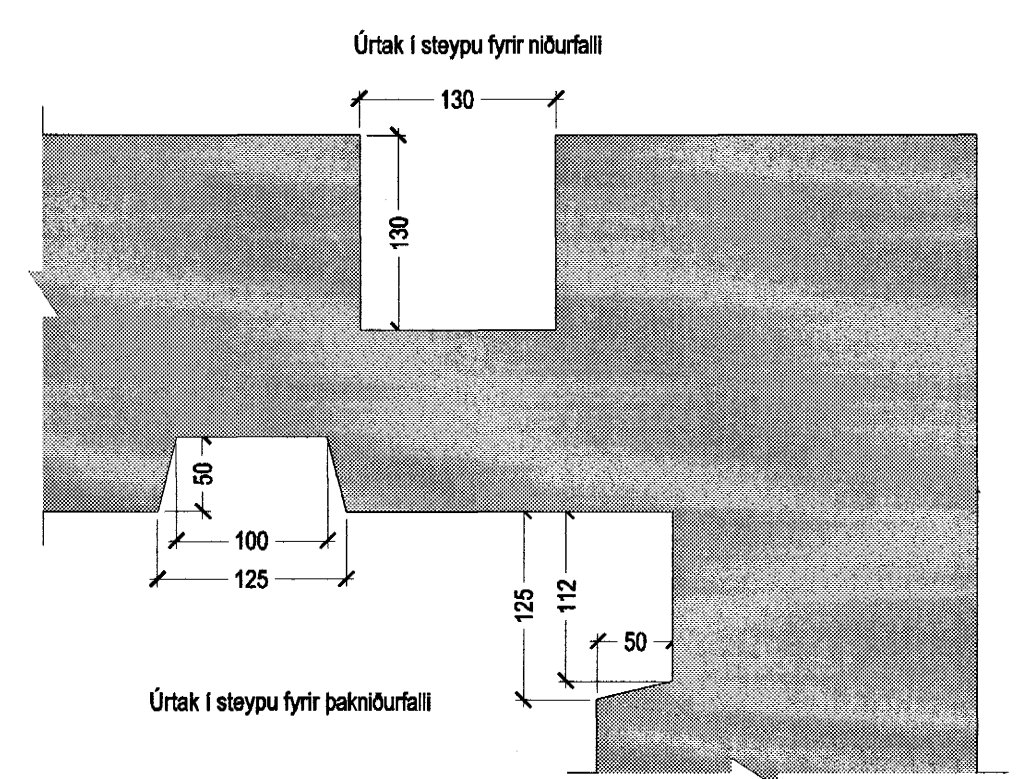
Lárétt prinsípeilli við úrtök í steypu mkv. 1:5
