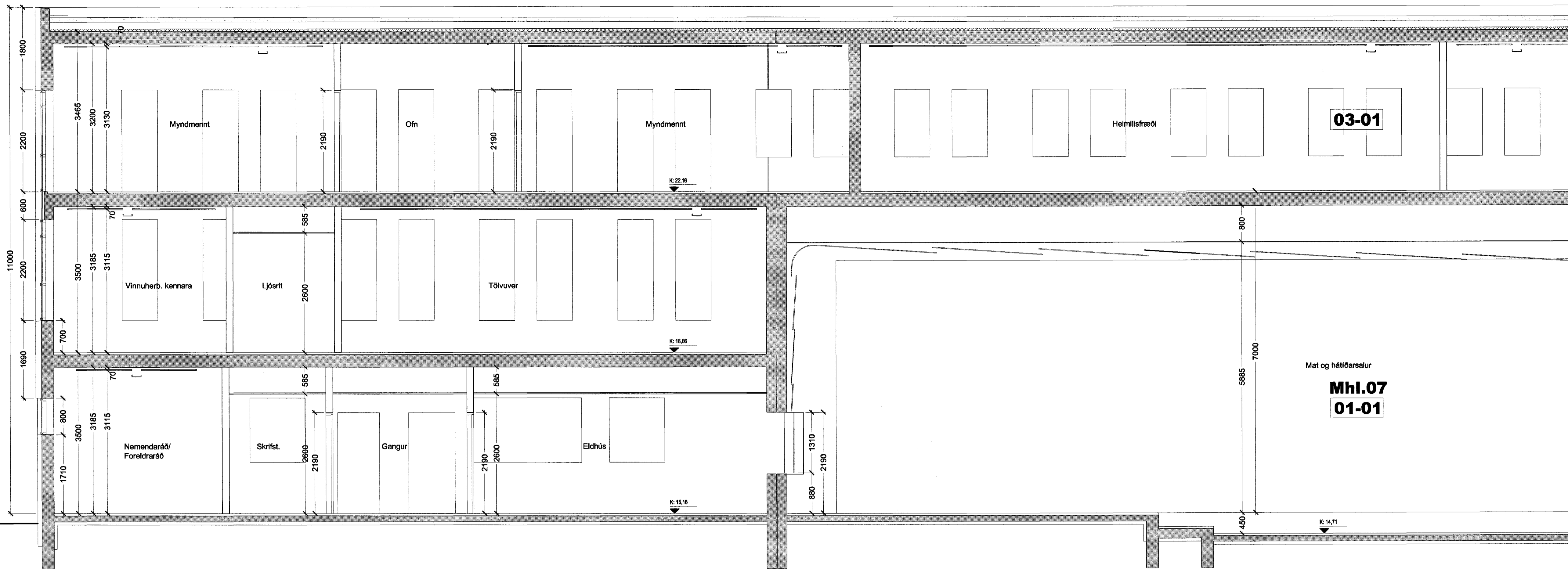
SNEIÐING 1 - 1
