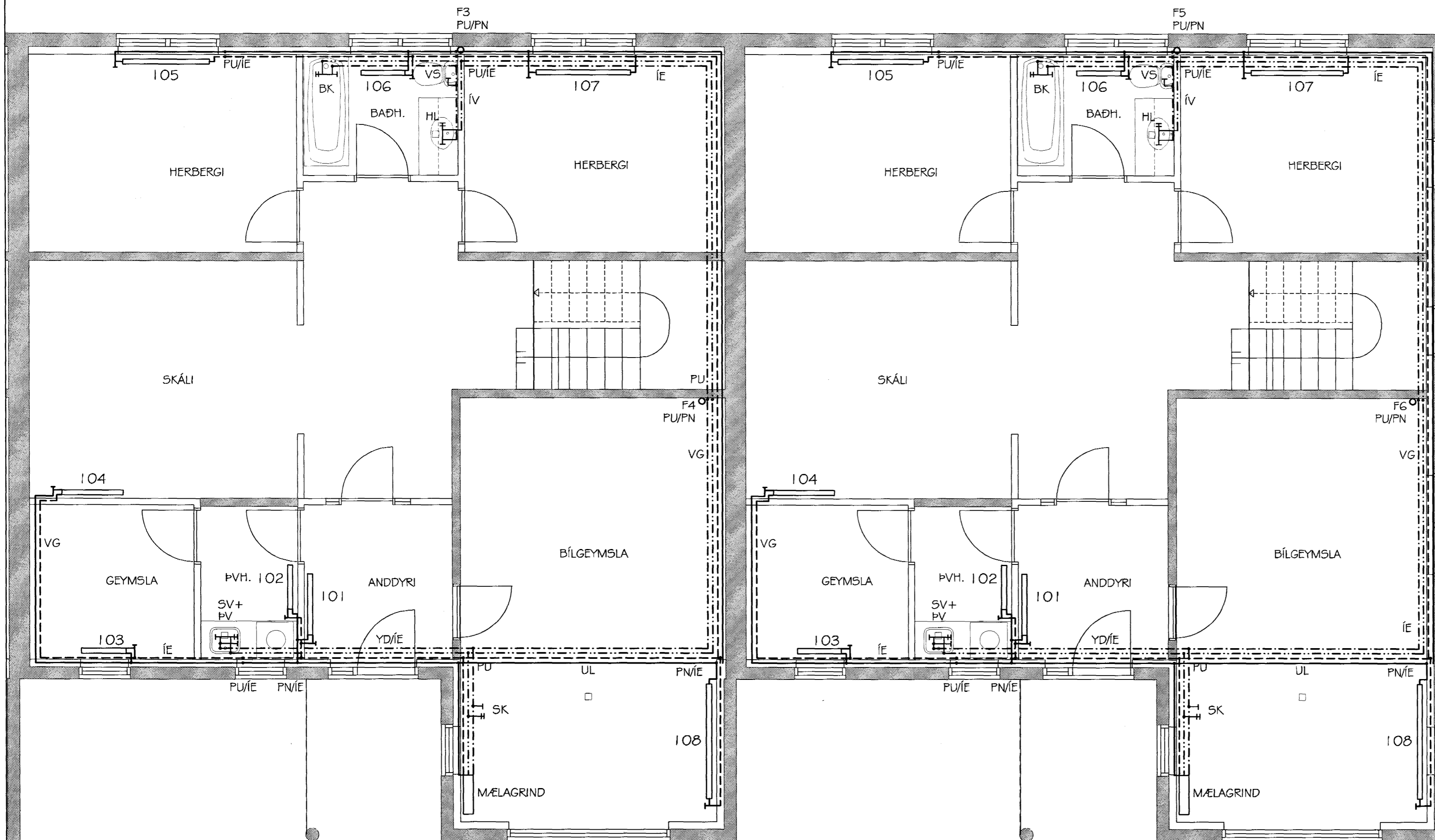
GAUKSÁS 15 NEYSLUVATNS- OG HITALAGNIR, FRÁRENNISLAGNIR GRUNNMYND NEDRI HÆÐAR MKV. 1:50
