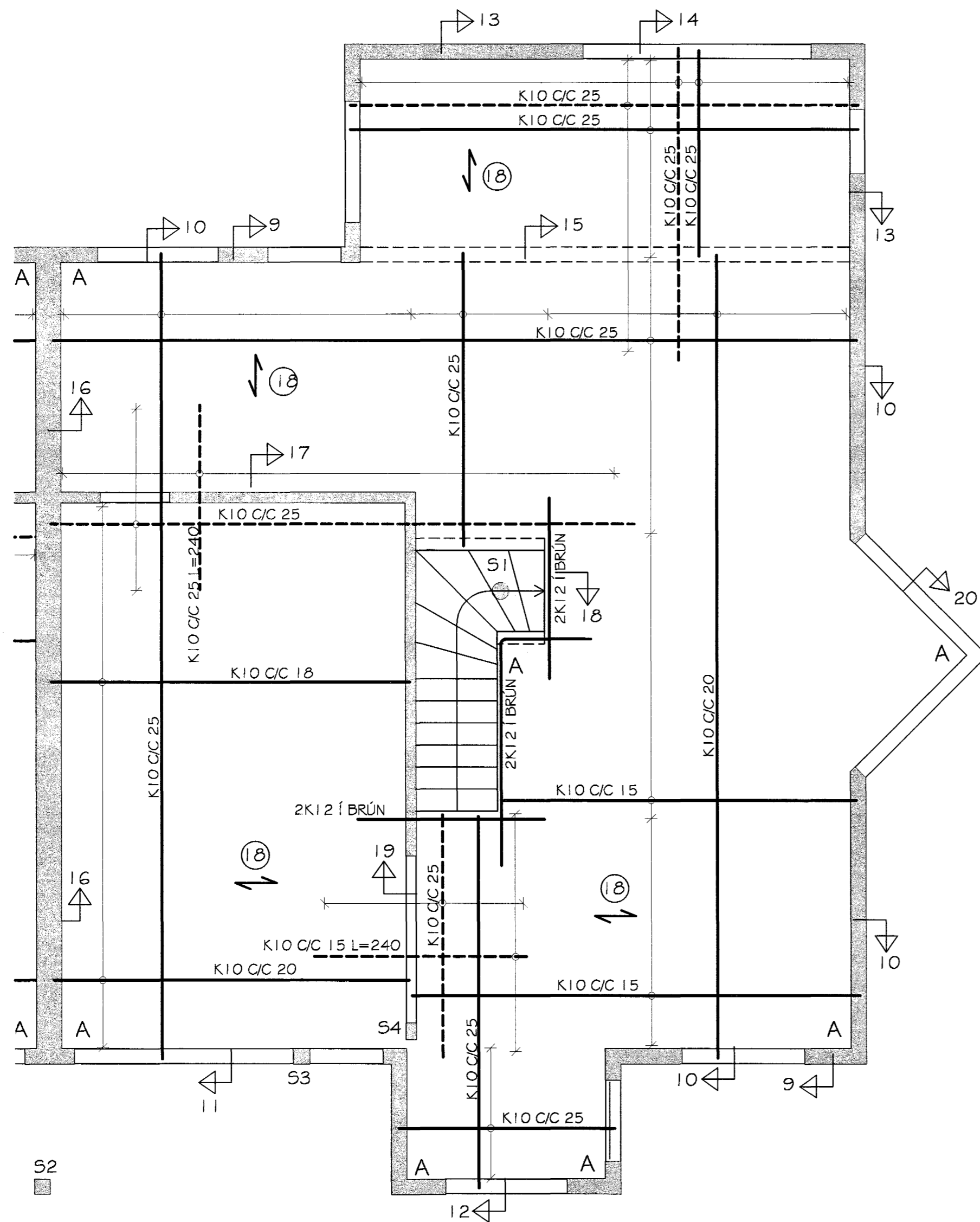
SVÖLUÁS 5 JÁRN Í PLÖTU YFIR 1. HÆÐ GRUNNMYND MKV. 1:50
