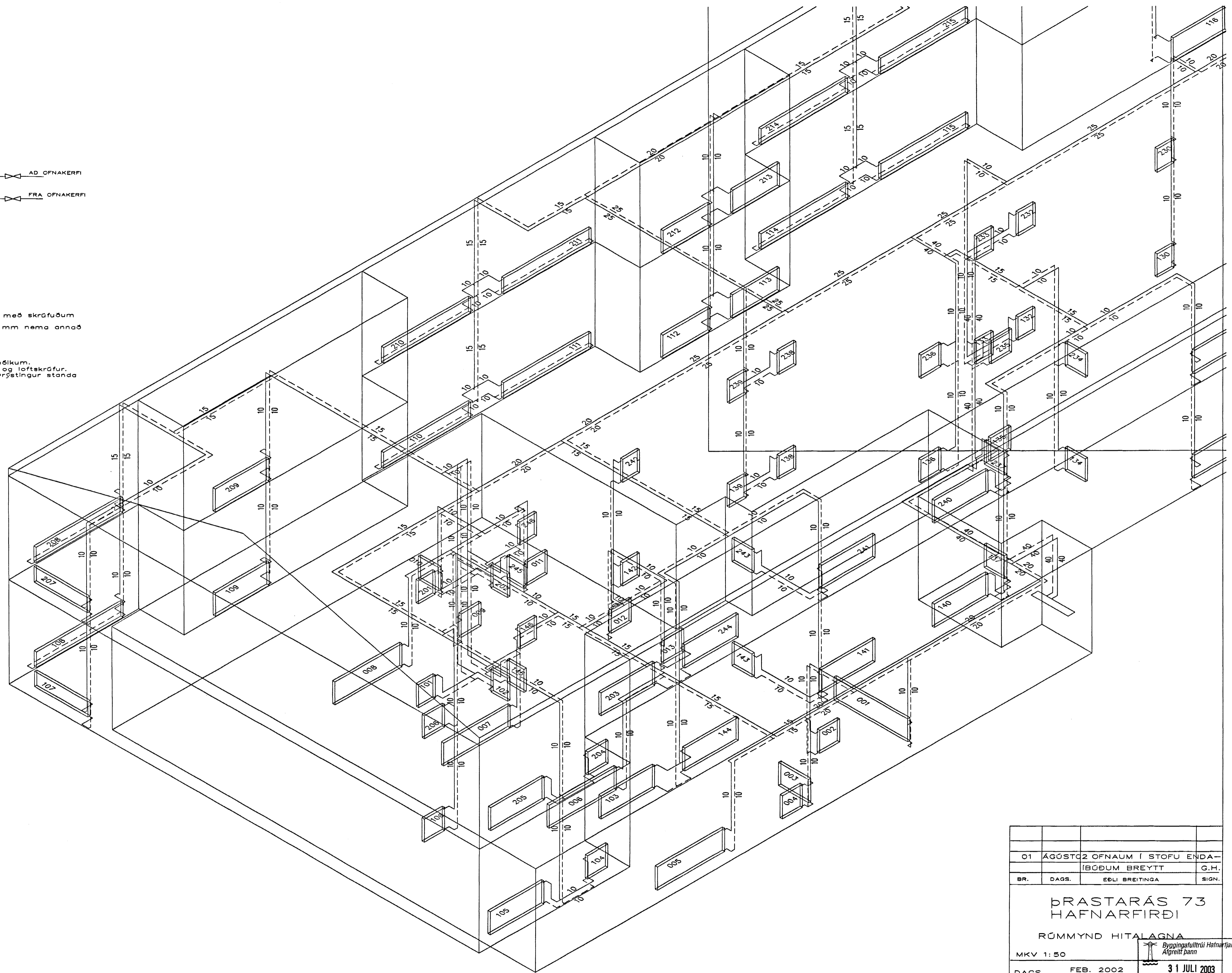
RÚMMYND HITALAGNA 1:50
