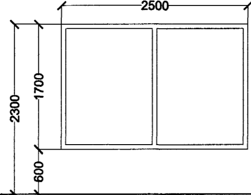
1 STK. STOFA
