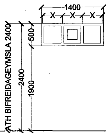
3 STK. BIFREIDAGEYMSLA
