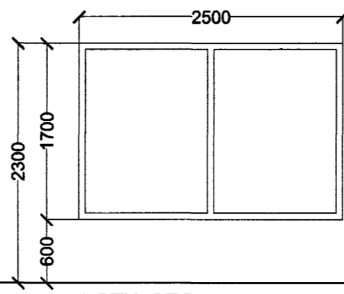
1 STK. STOFA
