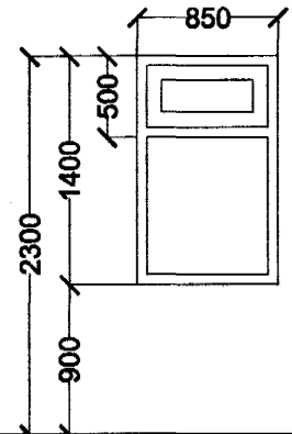
1 STK. ELDHÚS.
