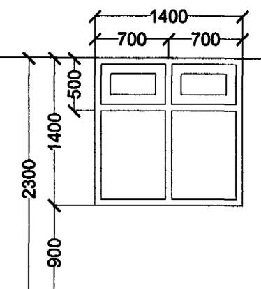
1 STK. ELDHÚS.
