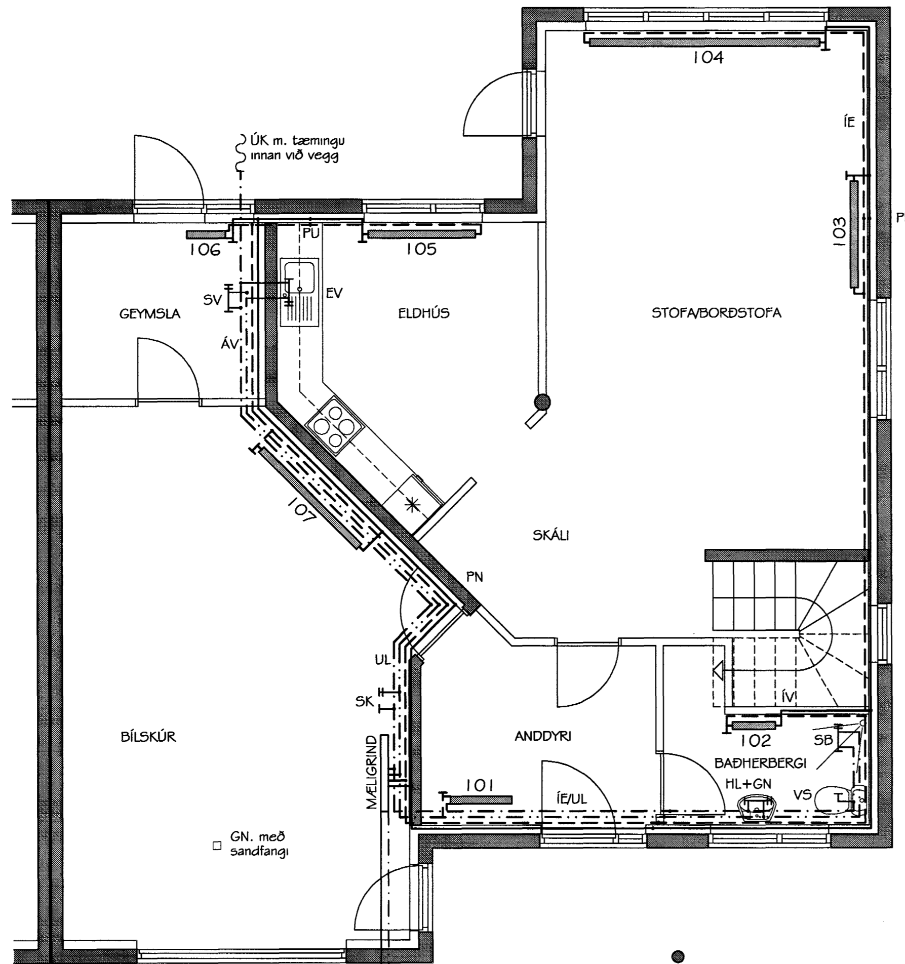
BLIKAÁS 30 HITA- OG NEYSLUVATNSLAGNIR GRUNNMYND NEDRI HÆÐAR MKV. 1:50
