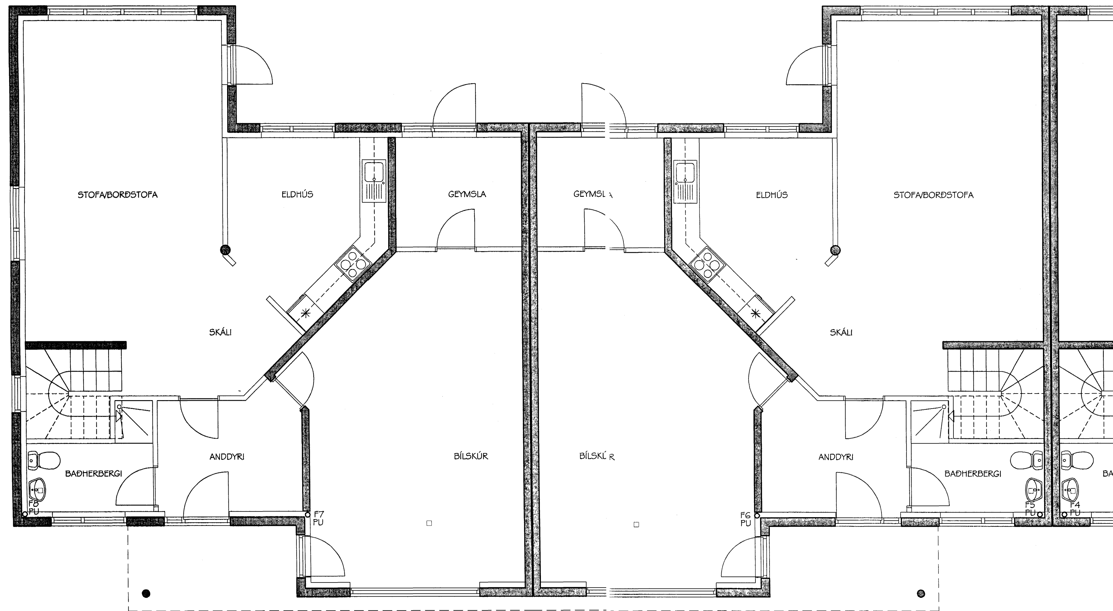
BLIKAÁS 34 OG 36 FRÁRENNISLAGNIR GRUNNMYND NEDRI HÆÐAR MKV. 1:50
