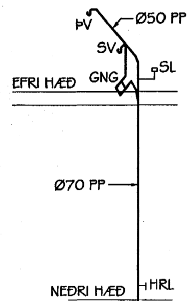
Fallstammi F5 mkv. 1:50
