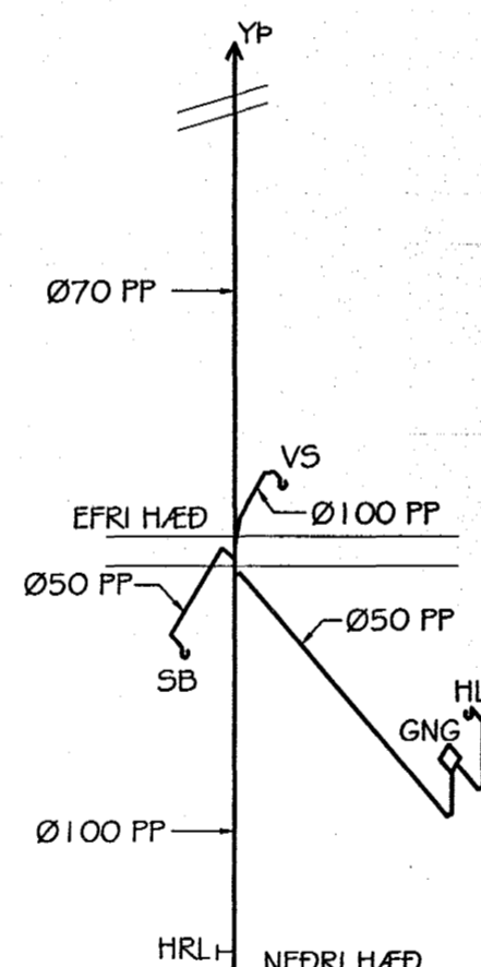
Fallstammi F7 mkv. 1:50
