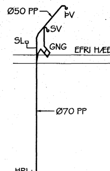
Fallstammi F8 mkv. 1:50
