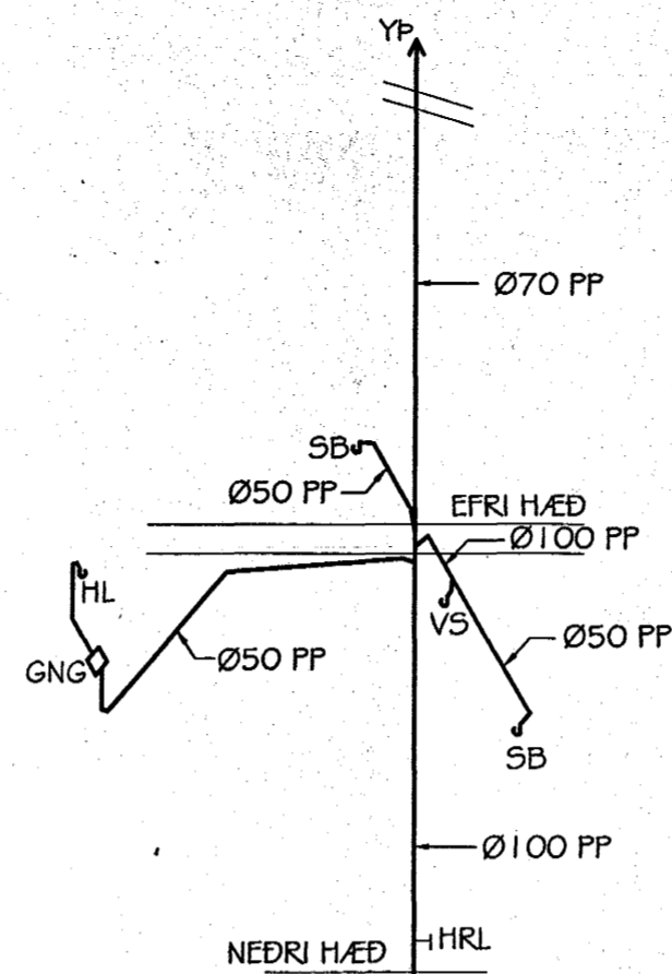
Fallstammi F3 mkv. 1:50
