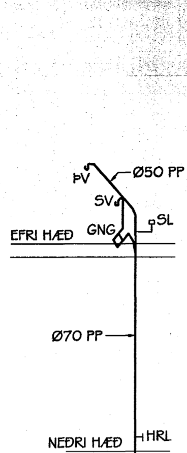
Fallstammi F1 mkv. 1:50
