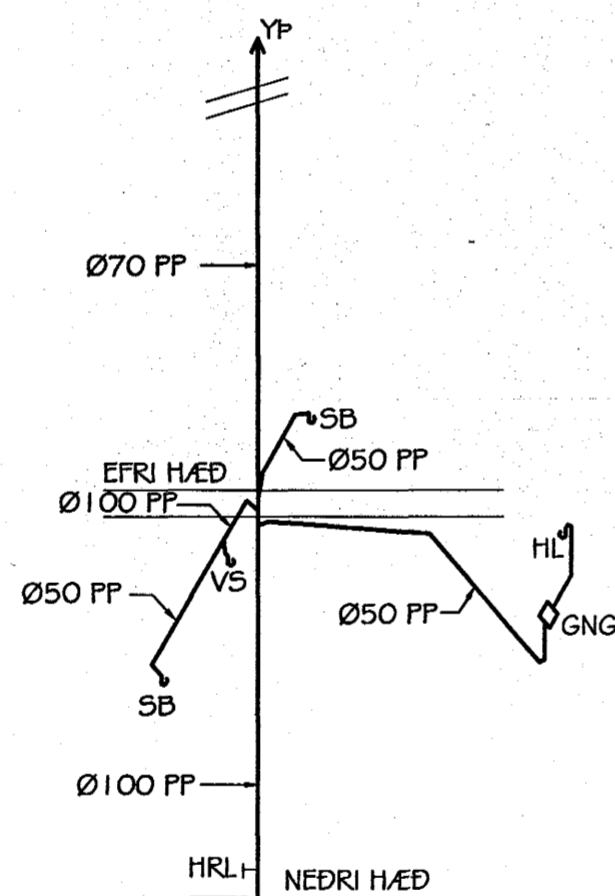
Fallstammi F6 mkv. 1:50
