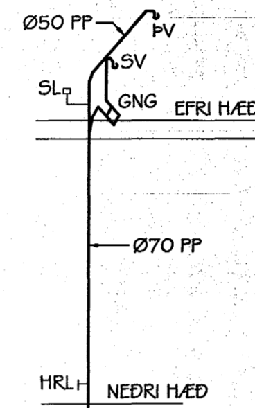
Fallstammi F4 mkv. 1:50
