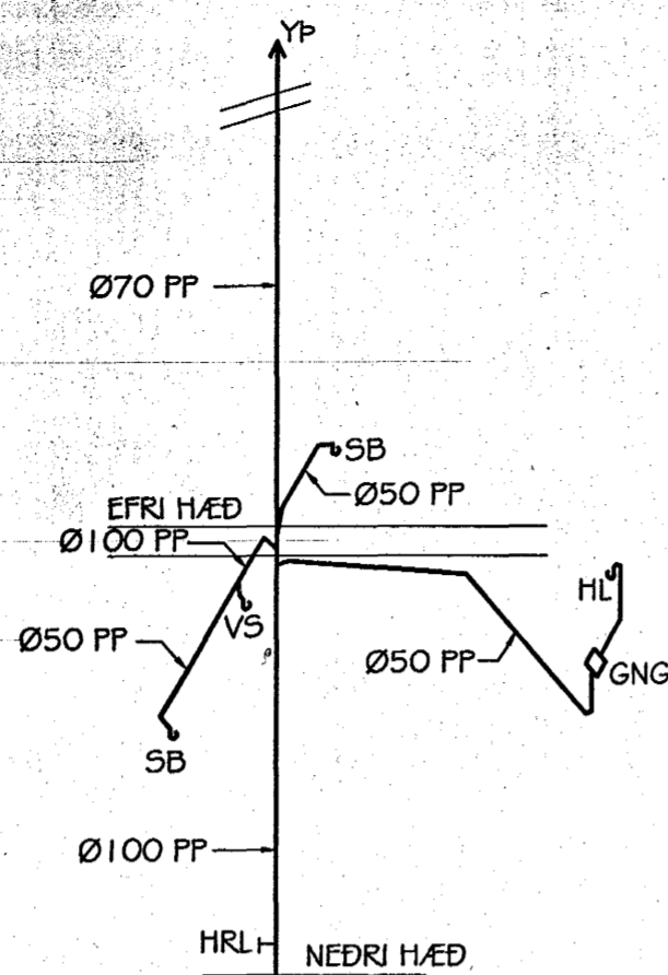
Fallstammi F2 mkv. 1:50
