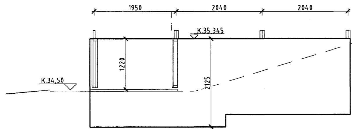
SKURÐUR A - A 1: 50
