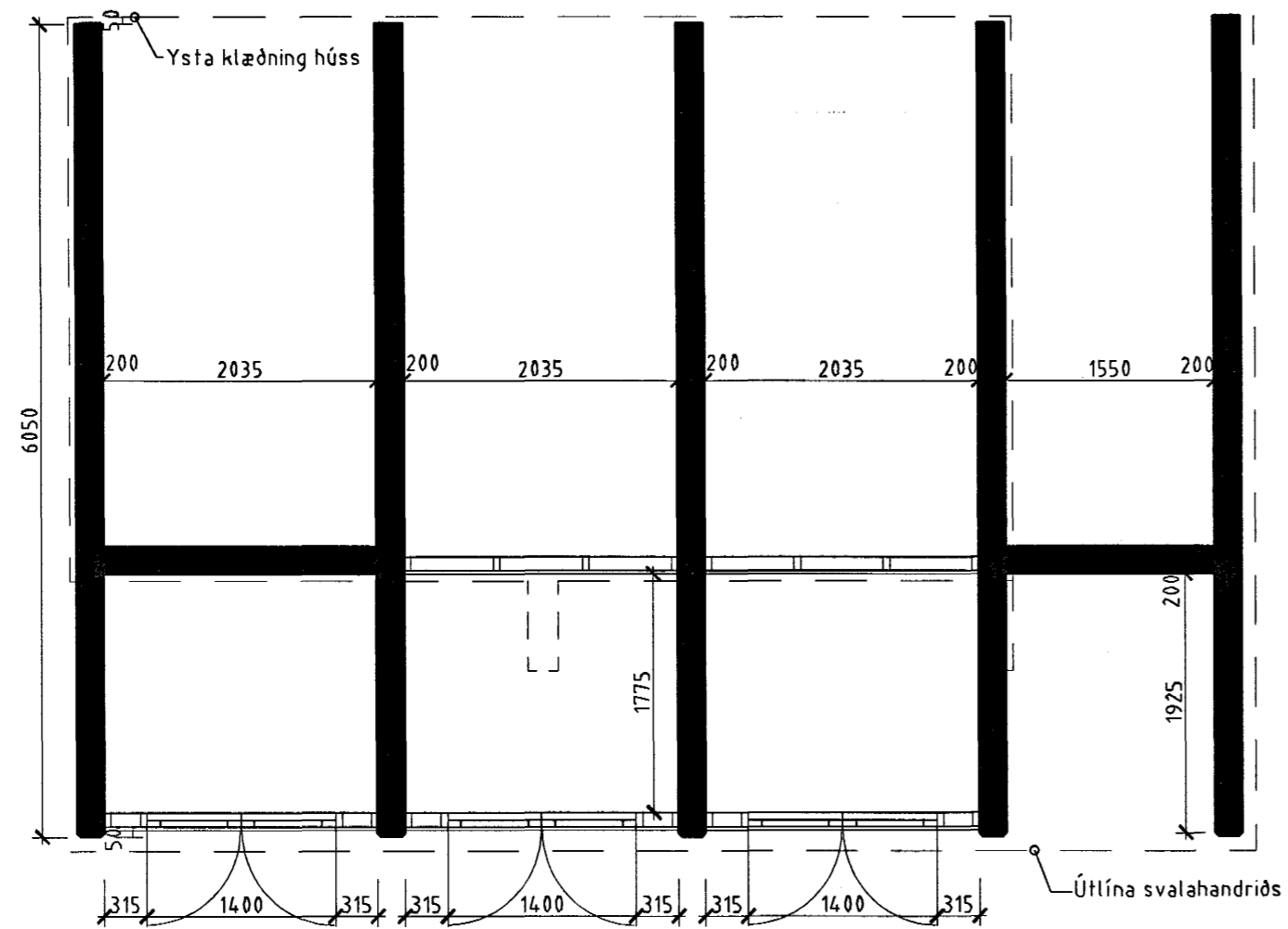
GRUNNMYND 1: 50
