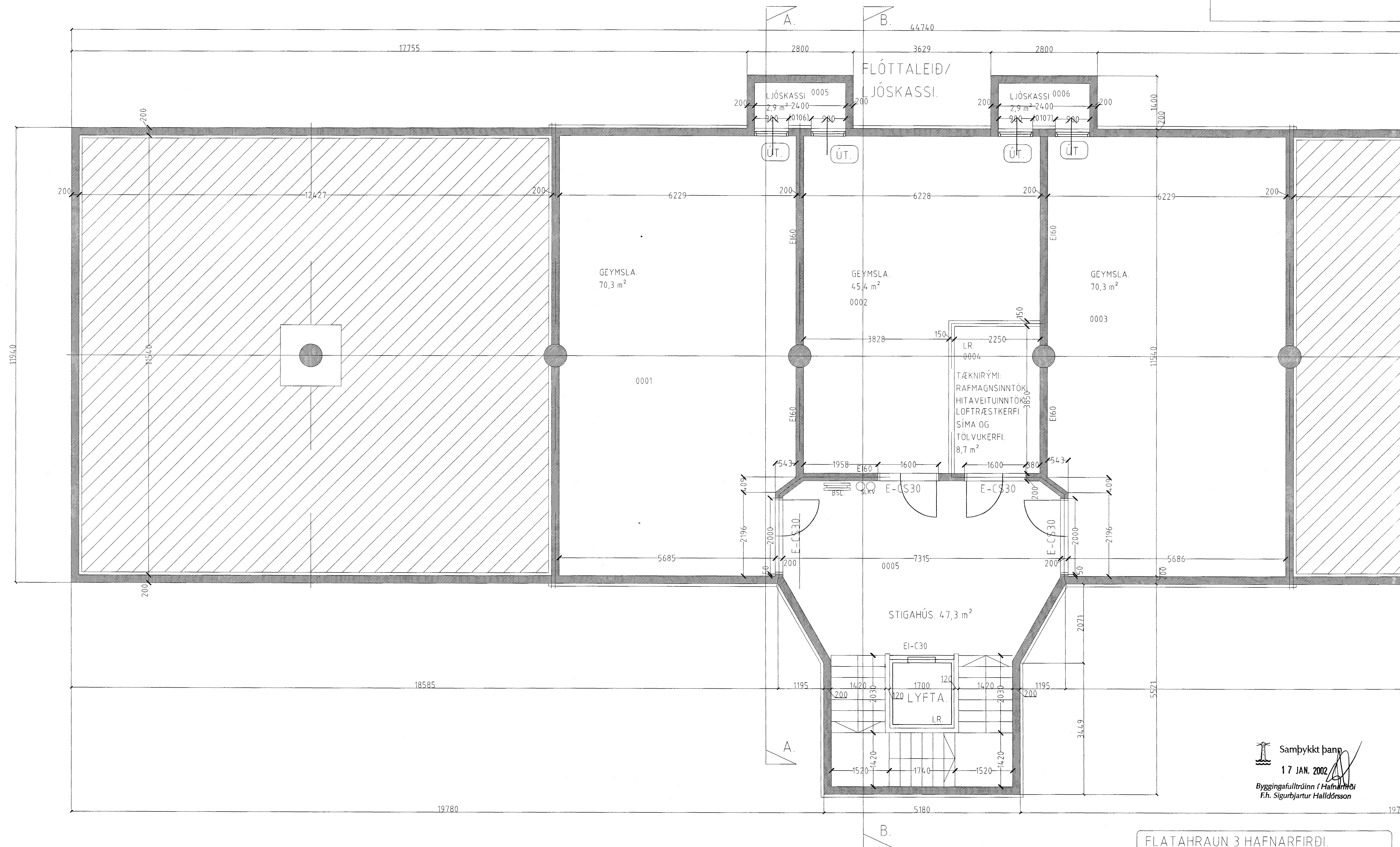
Grunnmynd kjallara. mkv. 1:50.
