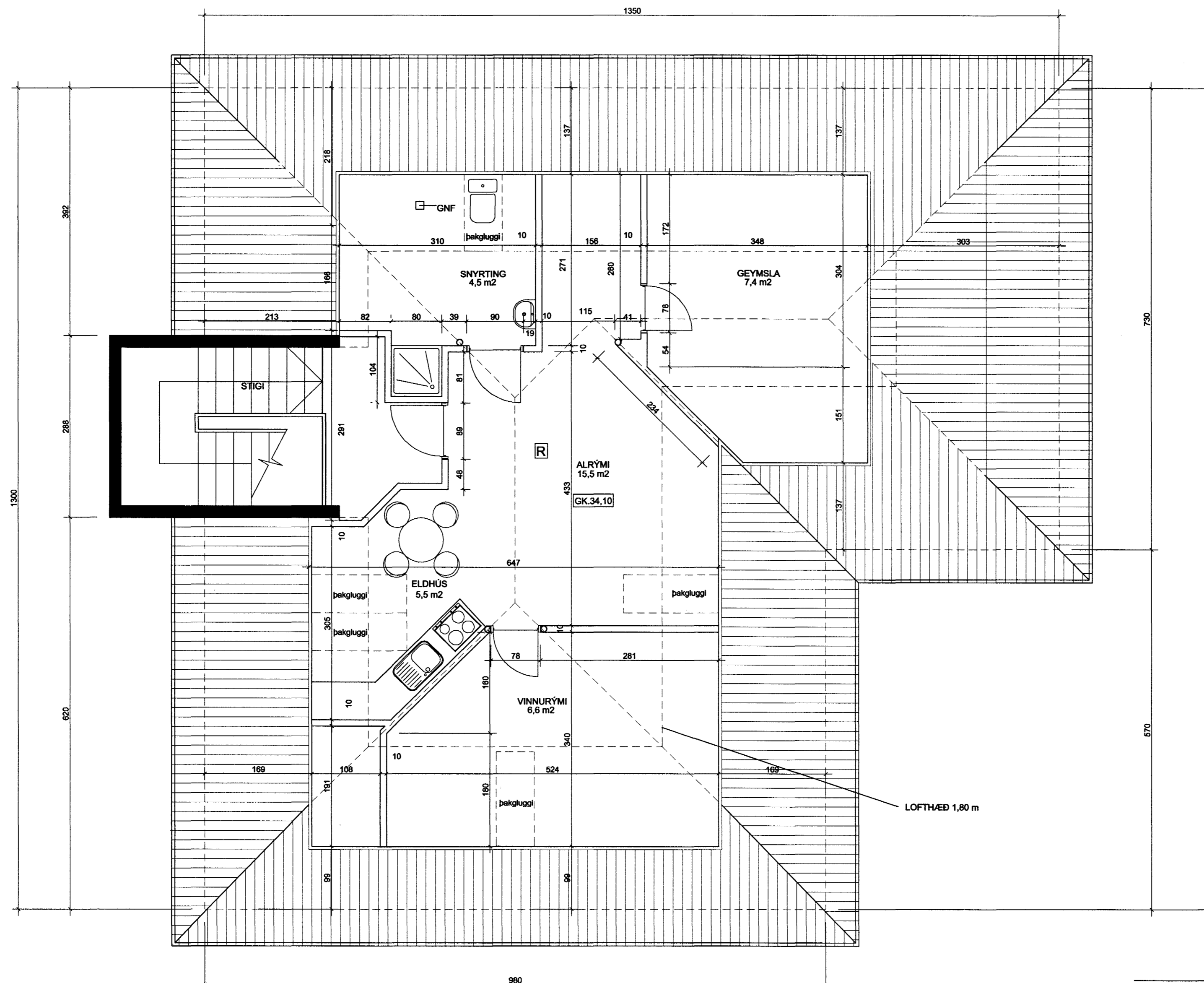
GRUNNMYND RISHÆÐAR 1:100
