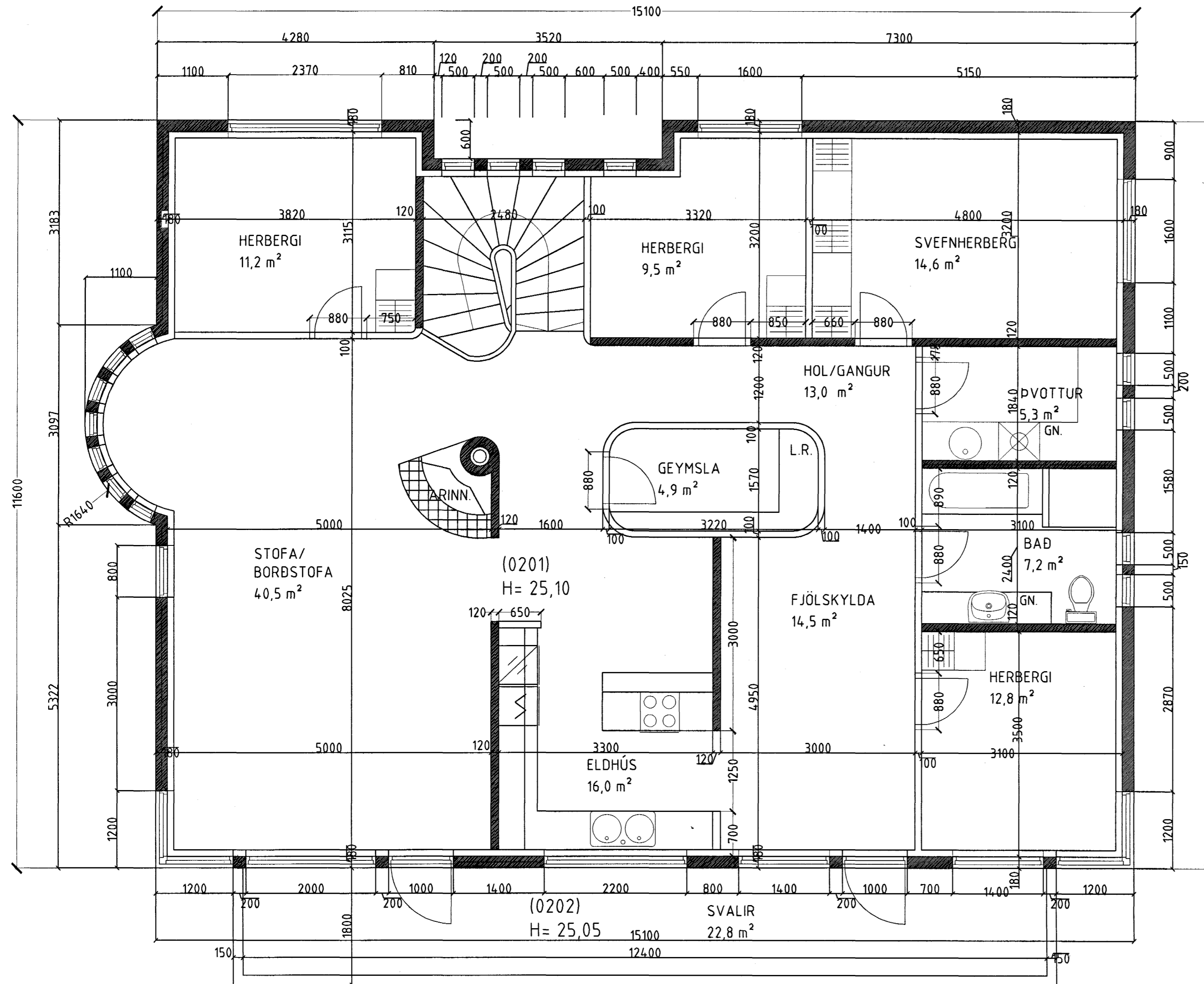
GRUNNMYND 2. HÆÐAR. MKV. 1:50.
