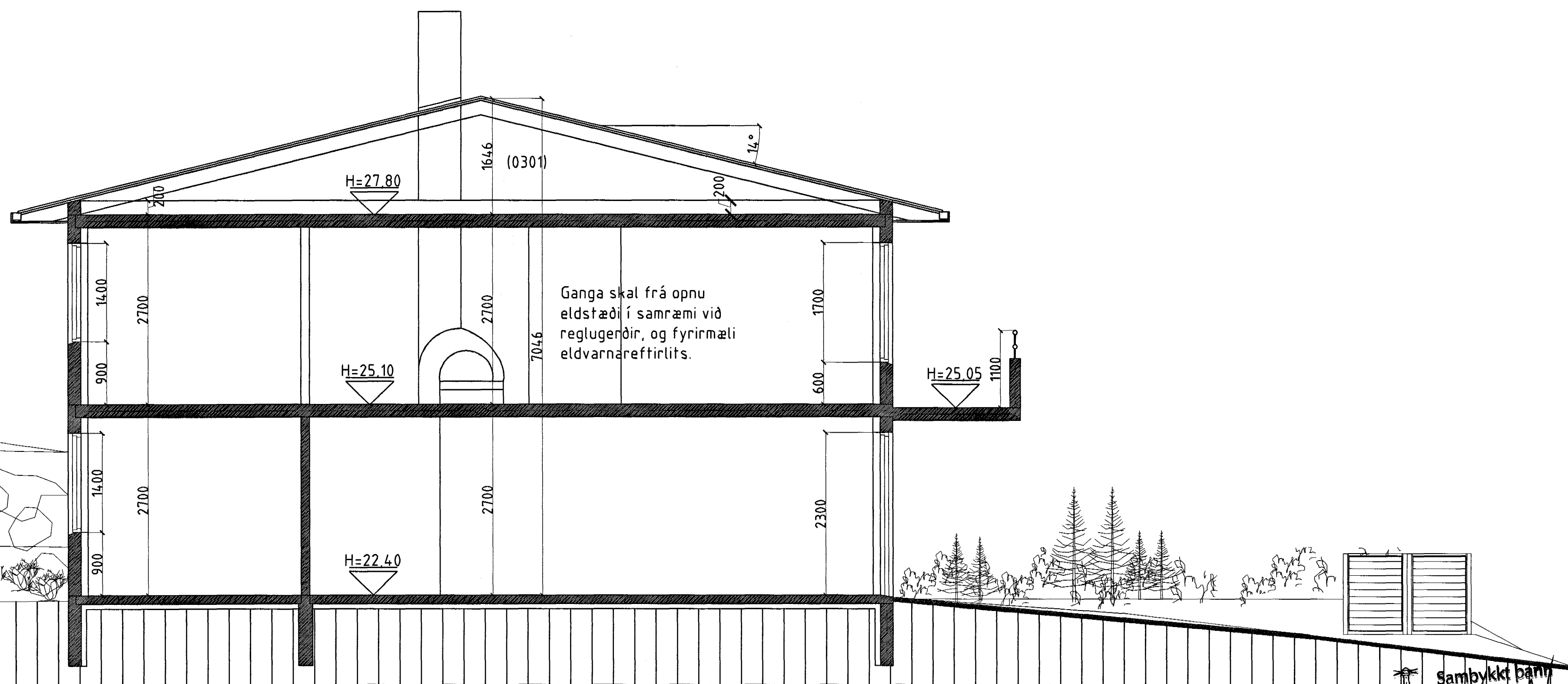
SNID B-B. MKV. 1:50.
