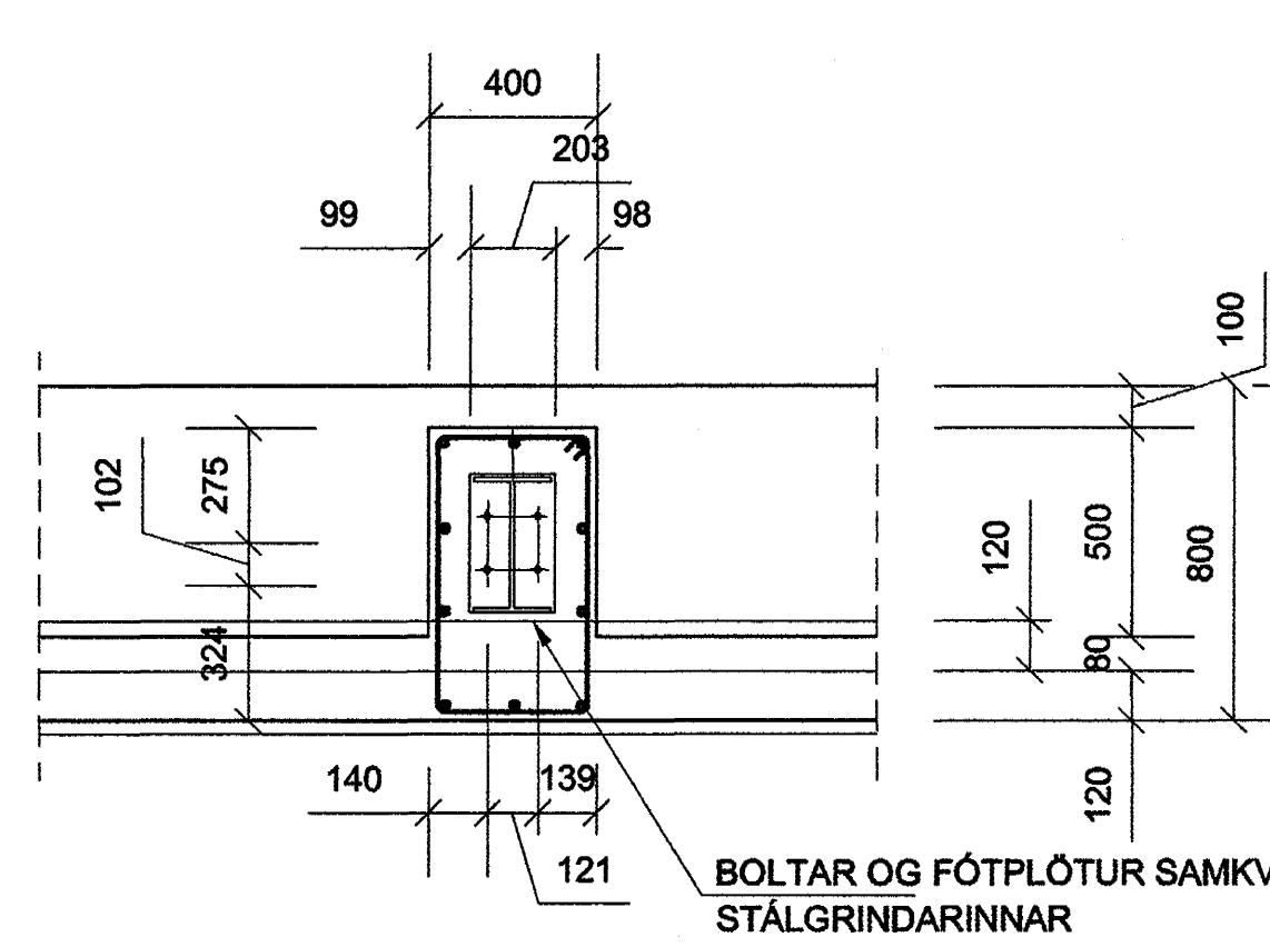
JÁRN Í SÚLUFÓTUM S4 OG STAÐSETNING FESTIBOLTA - GRUNNMYND - MKV. 1:20
