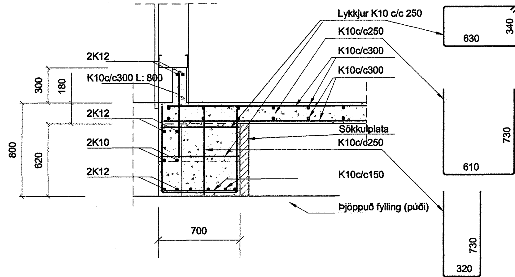
JÁRN Í SÚLUFÓTUM S6 - SNIÐ MKV. 1:20
