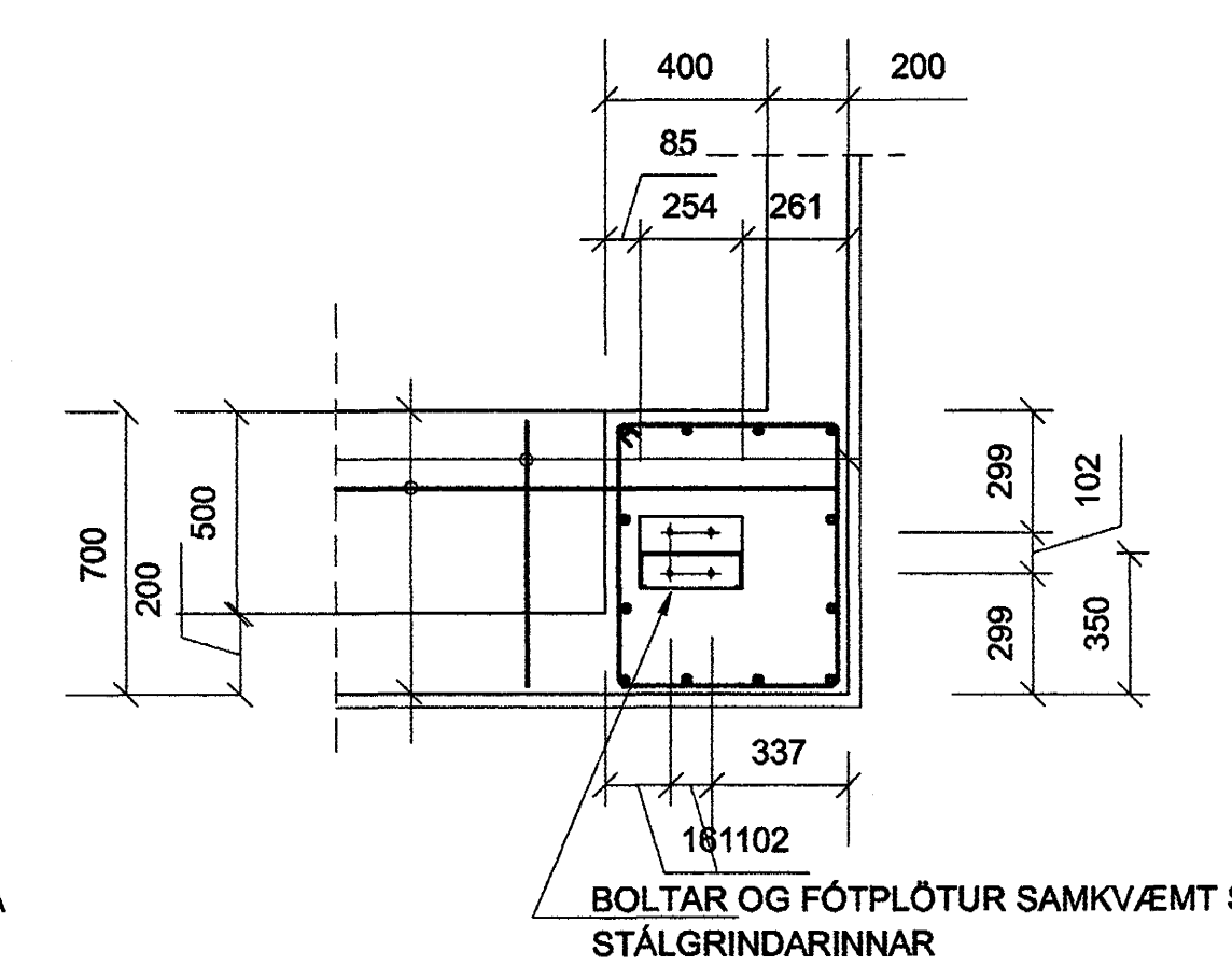
JÁRN Í SÚLUFÓTUM S9 OG STAÐSETNING FESTIBOLTA - GRUNNMYND - MKV. 1:20
