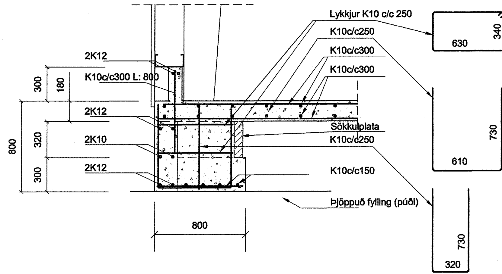
JÁRN Í SÚLUFÓTUM S4 OG S5 - SNIÐ MKV. 1:20
