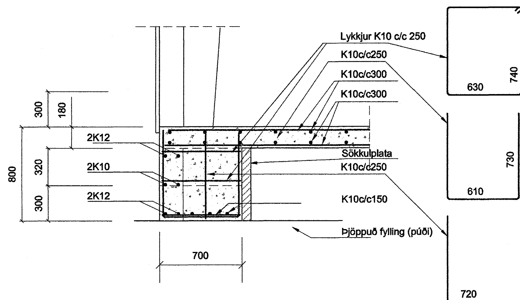
JÁRN Í SÚLUFÓTUM S8 - SNIÐ MKV. 1:20
