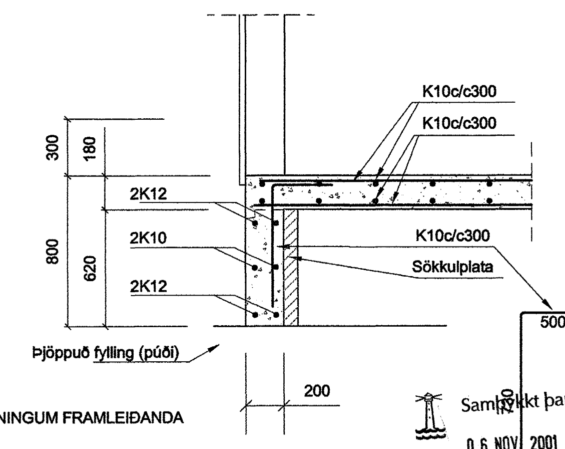
SNIÐ Í SÖKKULVEGGI GAFLA ÞJÓNUSUHÚSS MKV. 1:20
