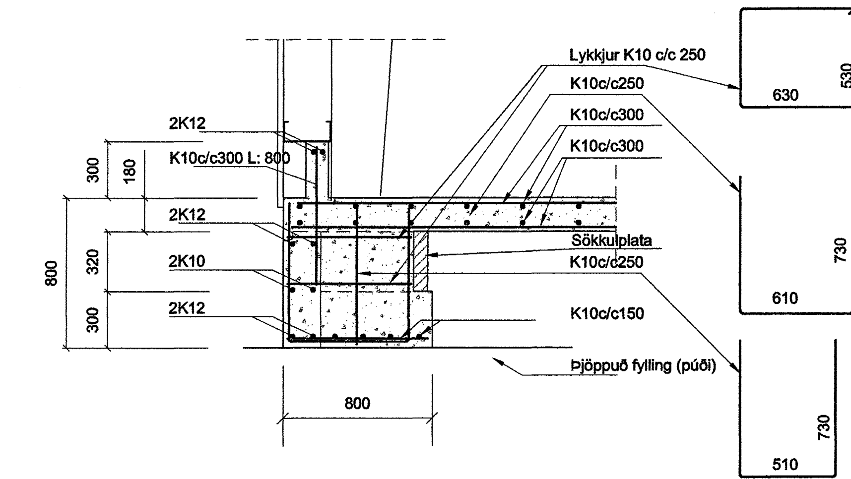
JÁRN Í SÚLUFÓTUM S9 - SNIÐ MKV. 1:20
