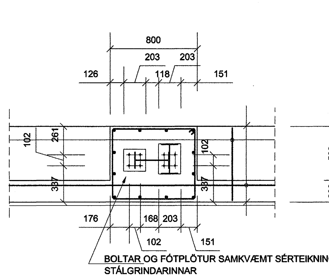
JÁRN Í SÚLUFÓTUM S8 OG STAÐSETNING FESTIBOLTA - GRUNNMYND - MKV. 1:20
