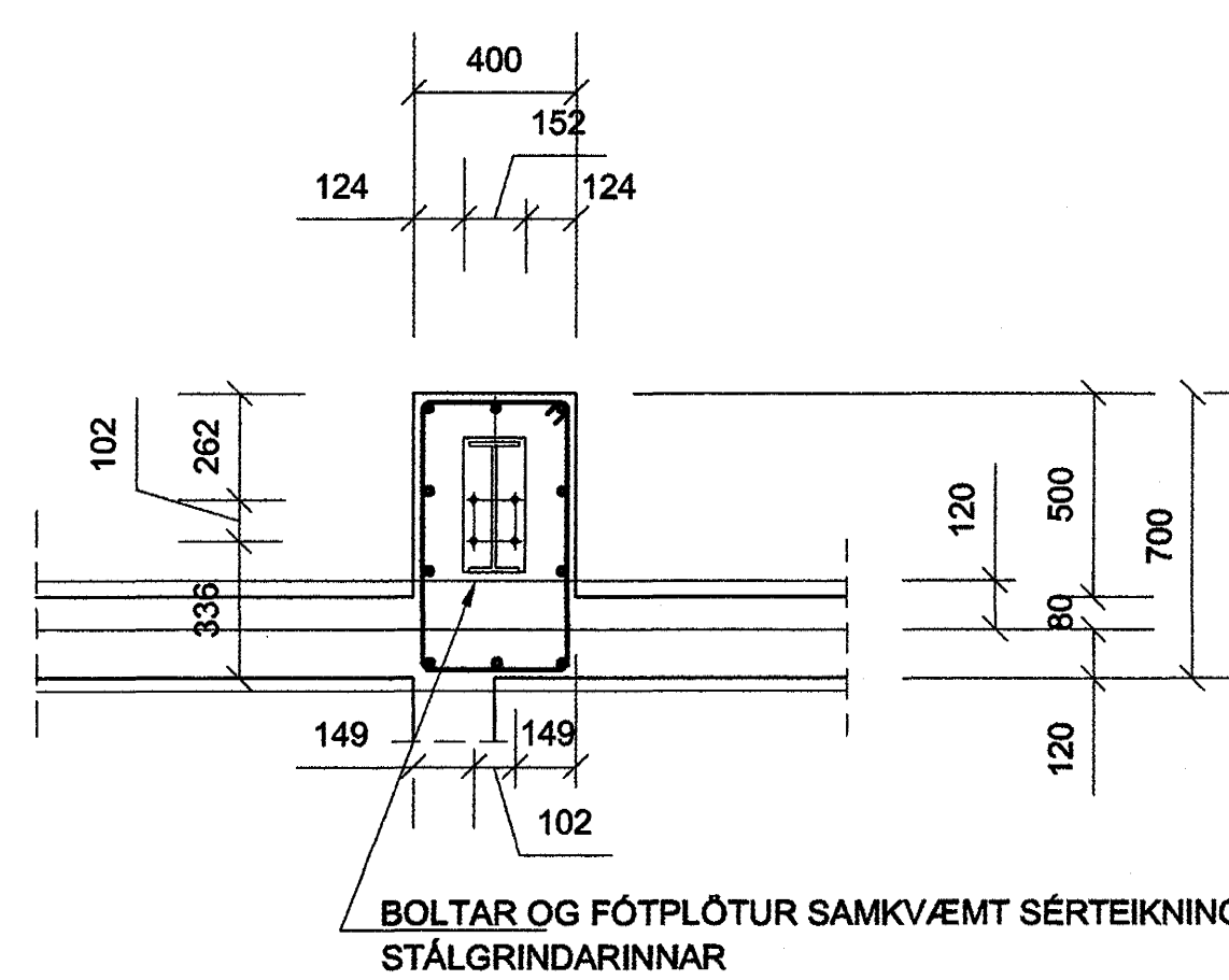
JÁRN Í SÚLUFÓTUM S6 OG STAÐSETNING FESTIBOLTA - GRUNNMYND - MKV. 1:20
