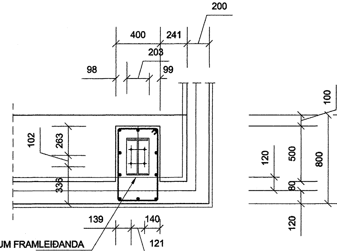
JÁRN Í SÚLUFÓTUM S5 OG STAÐSETNING FESTIBOLTA - GRUNNMYND - MKV. 1:20
